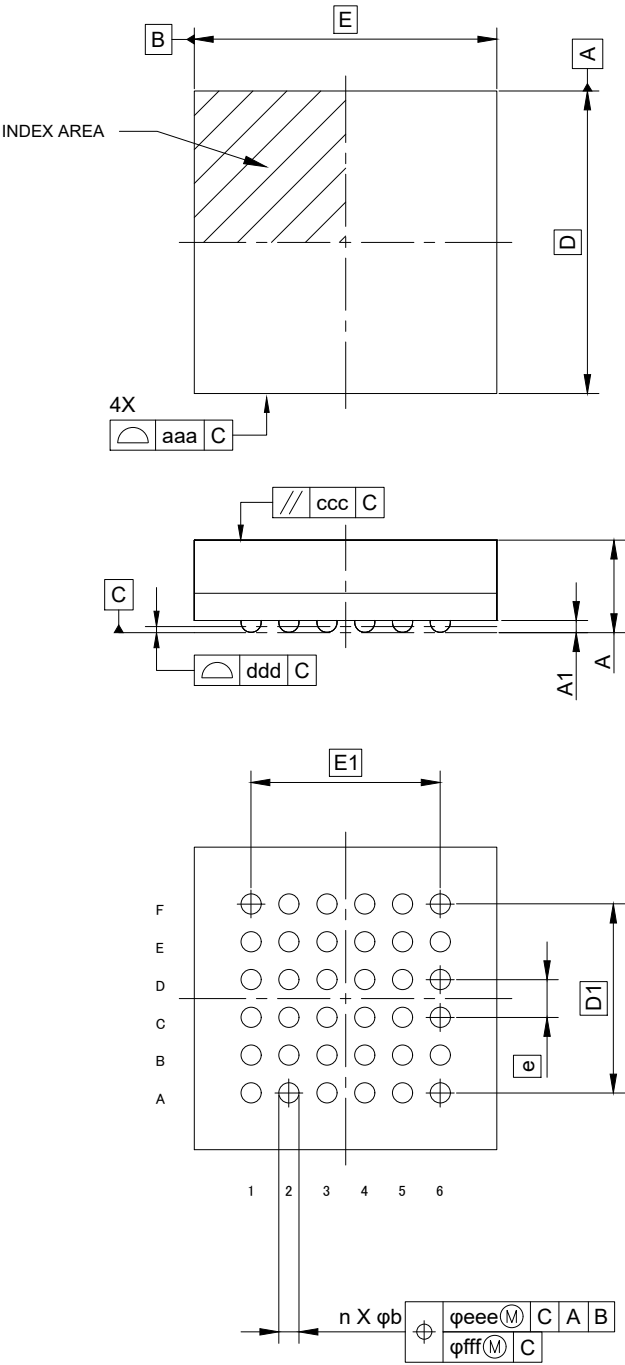
図 A2.5 BGA 36 ピン
