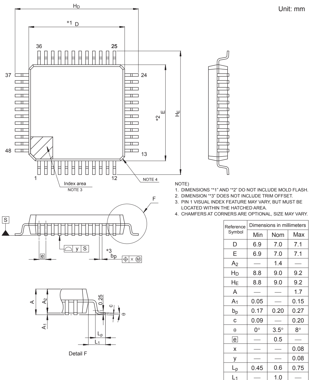
図 A2.5 LQFP 48 ピン (1)
