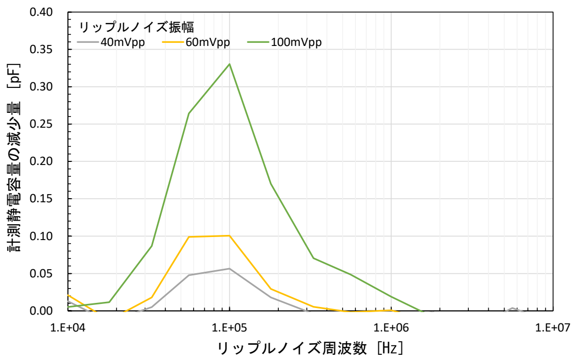
図 2.47 計測静電容量の減少量
