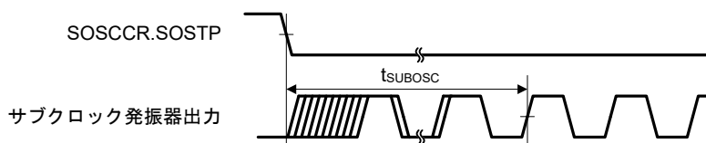
図 2.6 サブクロック発振開始タイミング
