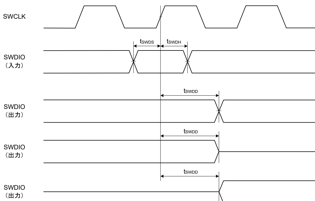
図 2.50 SWD 入出力タイミング
