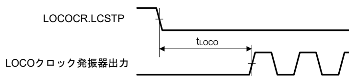
図 2.4 LOCO クロック発振開始タイミング
