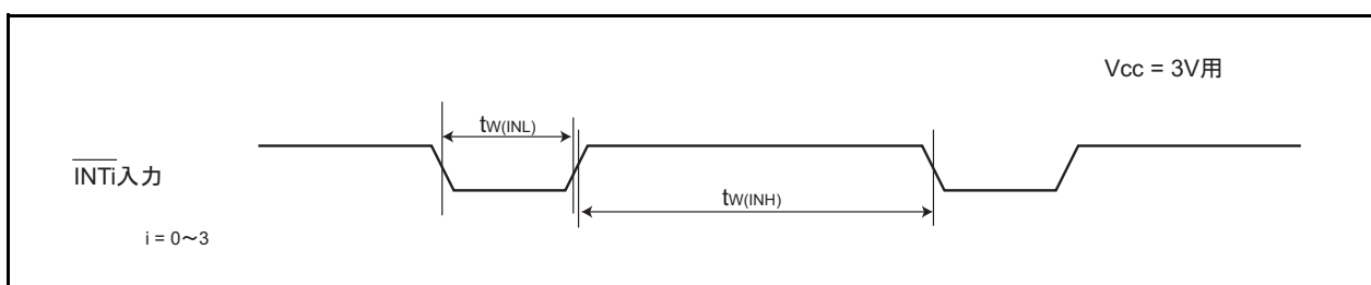
図5.15 Vcc=3V時の外部割り込み \overline{\text{INTi}} 入力タイミング (i=0 ~ 3)
