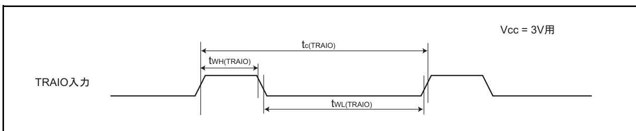
図5.13 V_{CC}=3V 時のTRAIO入力タイミング
