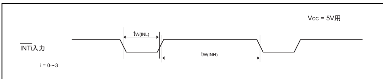
図5.11 V_{cc}=5V 時の外部割り込み \overline{\text{INT}}_i 入力タイミング ( i=0 \sim 3 )
