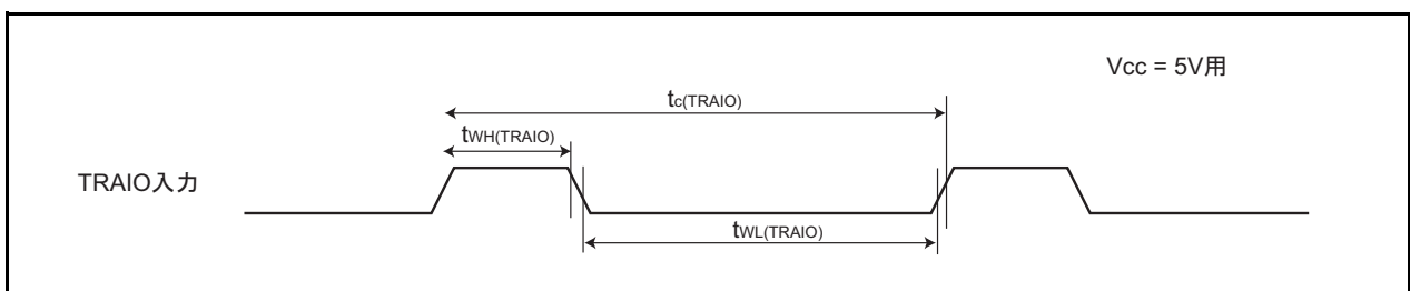
図5.9 V_{CC}=5V 時のTRAIO入力タイミング
