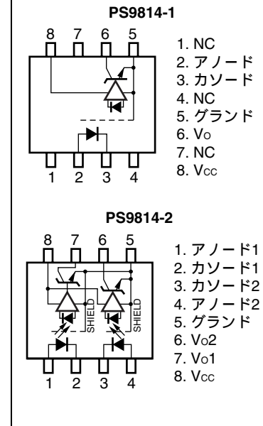
端子接続図 (Top View)
