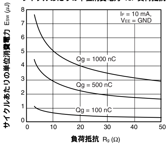
サイクルあたりの単位消費電力 vs. 負荷抵抗
