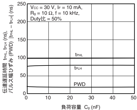
伝達遅延時間, パルス幅ひずみ vs. 負荷容量
