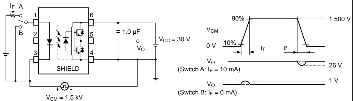
图9 CMR 測定回路と波形
