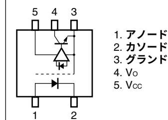
端子接続図 (Top View)
