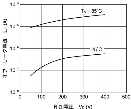
オフ・リーク電流 vs. 印加電圧
