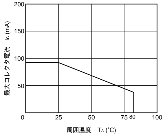
最大コレクタ電流 vs. 周囲温度
