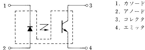
端子接続（Bottom View）
