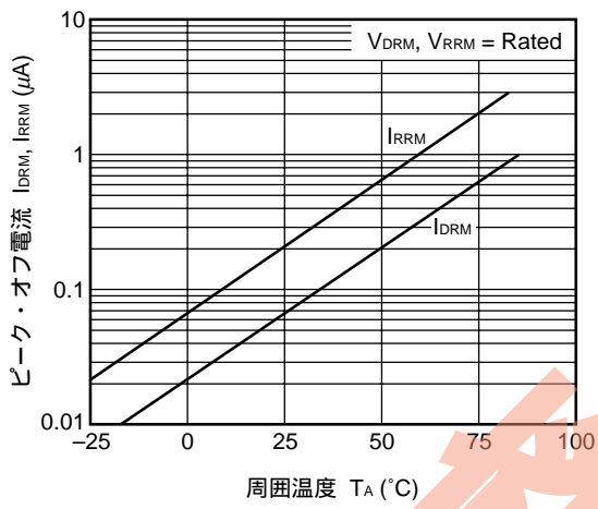
ピーク・オフ電流 vs. 周囲温度
