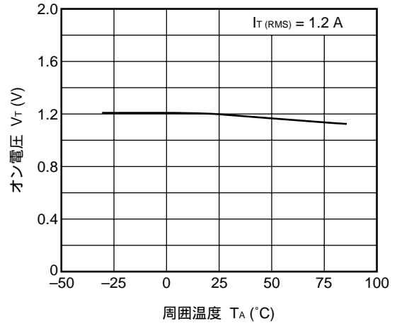
オン電圧 vs. 周囲温度
