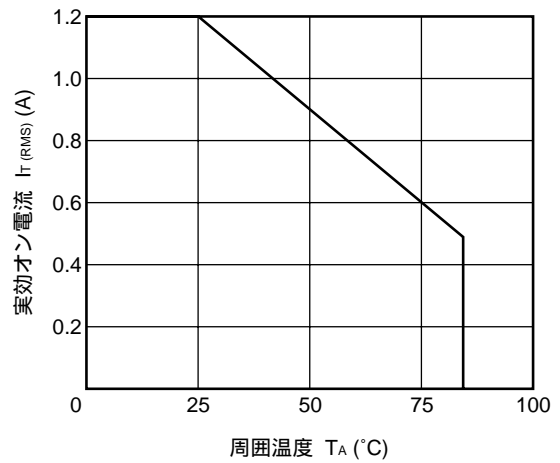
実効オン電流 vs. 周囲温度
