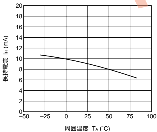
保持電流 vs. 周囲温度
