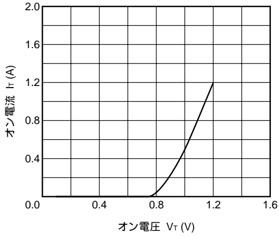
オン電流 vs. オン電圧
