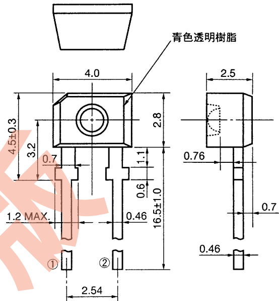
端子接続
