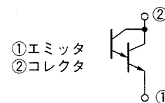
端子接続
