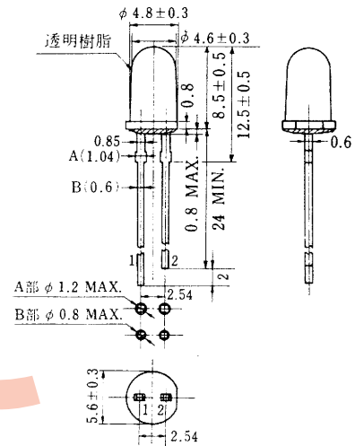
外形図 (Unit : mm)
