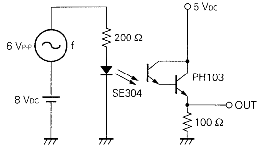
周波数応答特性測定回路
