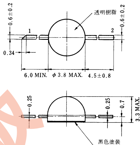
電極接続 1. コレクタ 2. エミッタ
