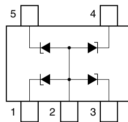
端子接続図
