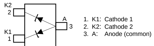
端子接続図
