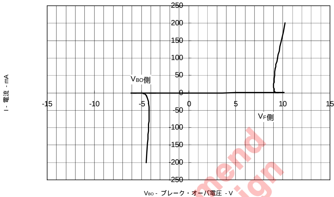
図1 I vs. V BO 特性例
