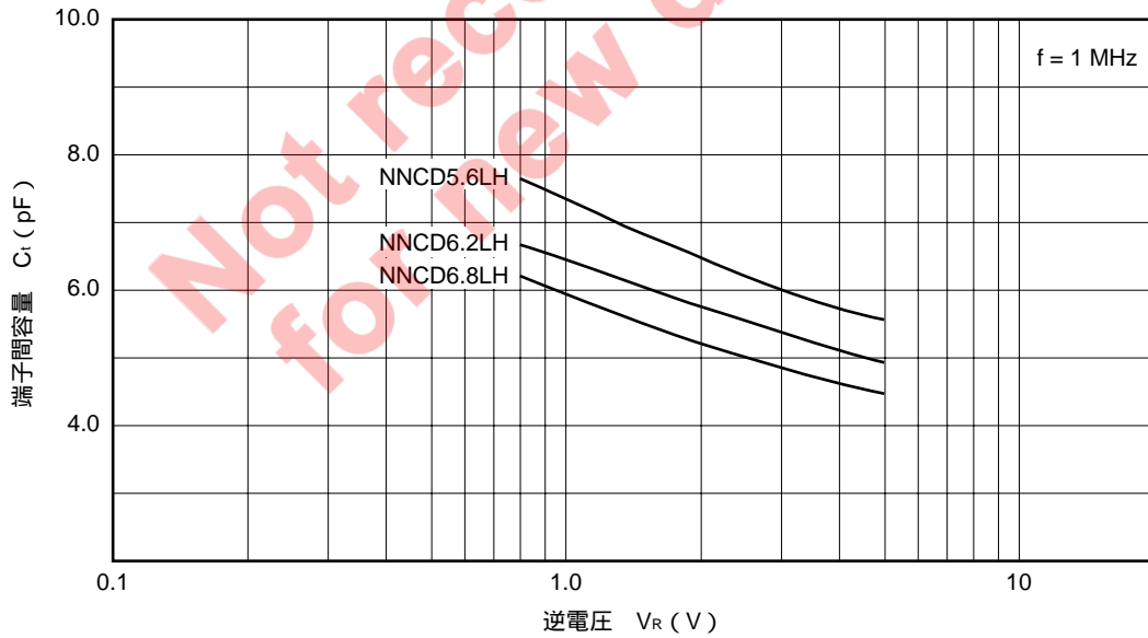
図3 C t -V R 特性例 (f = 1 MHz)
