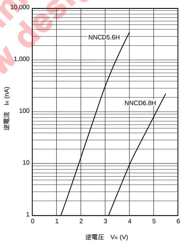
図3 I_R - V_R 特性例
