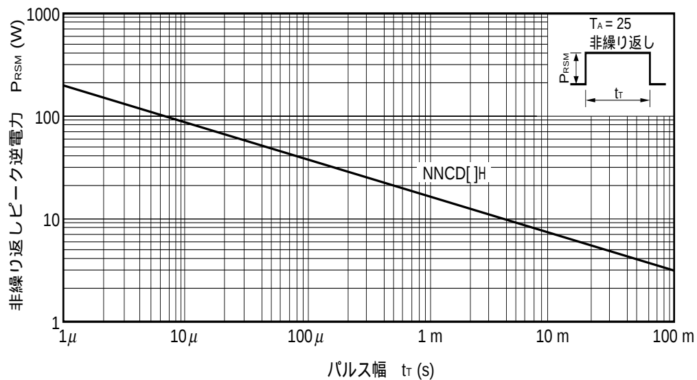
図6 サージ逆電力定格
