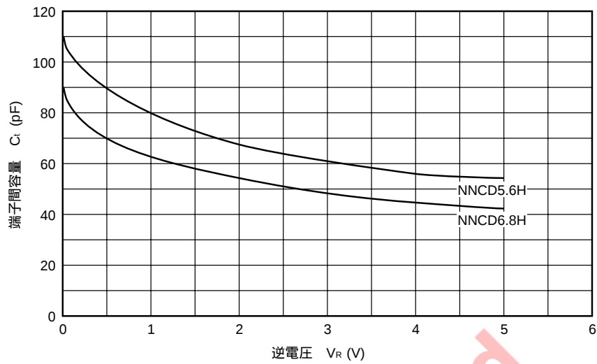
図4 C_t - V_R 特性例
