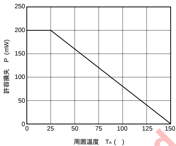
図1 P - T_A 定格
