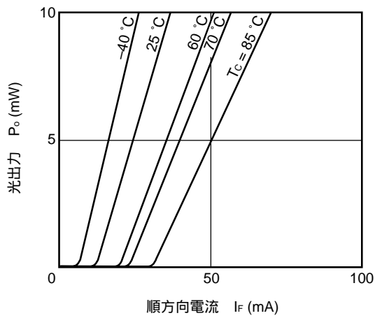
光出力 対 順方向電流
