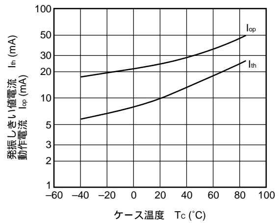
発振しきい値電流, 動作電流 対 ケース温度
