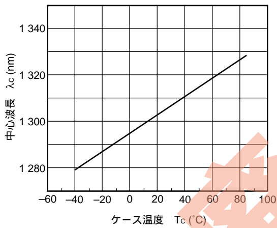
中心波長 対 ケース温度
