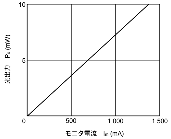
光出力 対 LDモニタ電流
