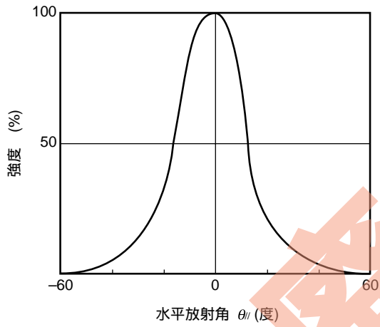
ファール・フィールド・パターン ( \theta_H )
