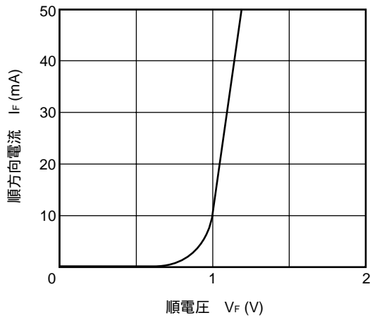
順方向電流 対 順電圧
