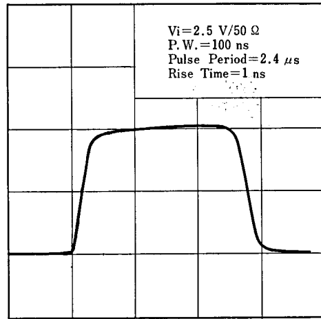
応答特性
