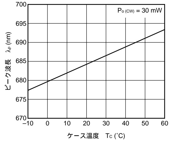
ピーク波長 vs. ケース温度
