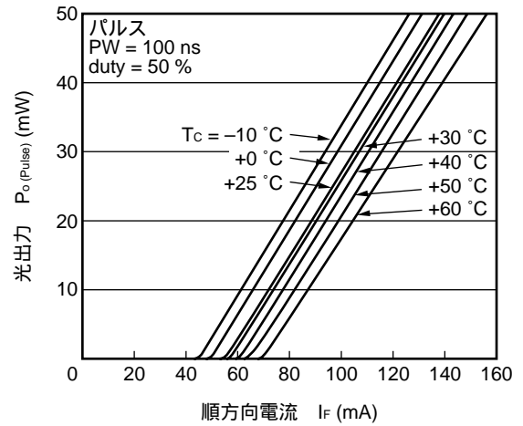
光出力 vs. 順方向電流
