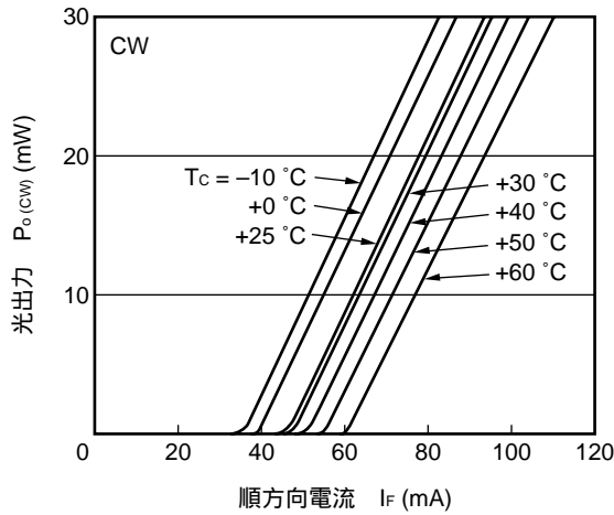
光出力 vs. 順方向電流
