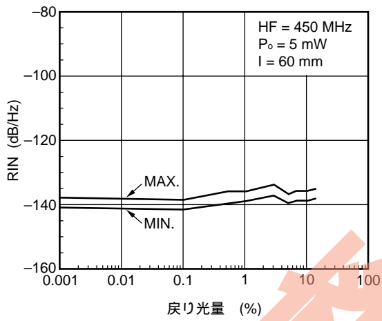
RIN特性
