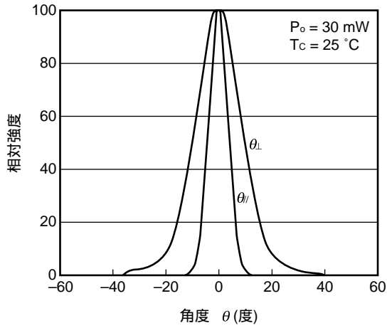
ファー・フィールド・パターン
