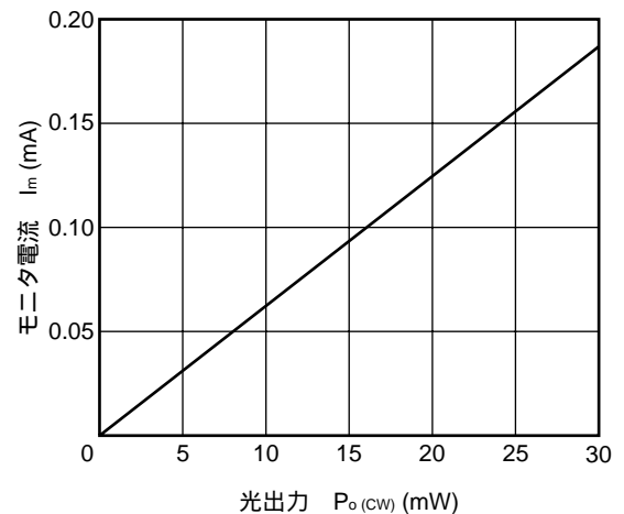
モニタ電流 vs. 光出力
