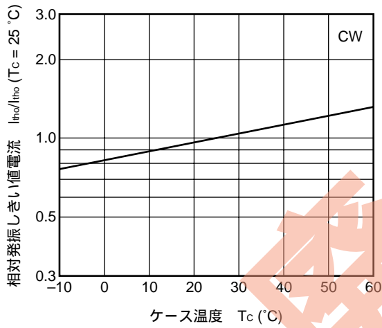
相対発振しきい値電流 vs. ケース温度
