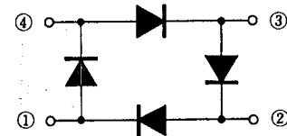
端子接続
