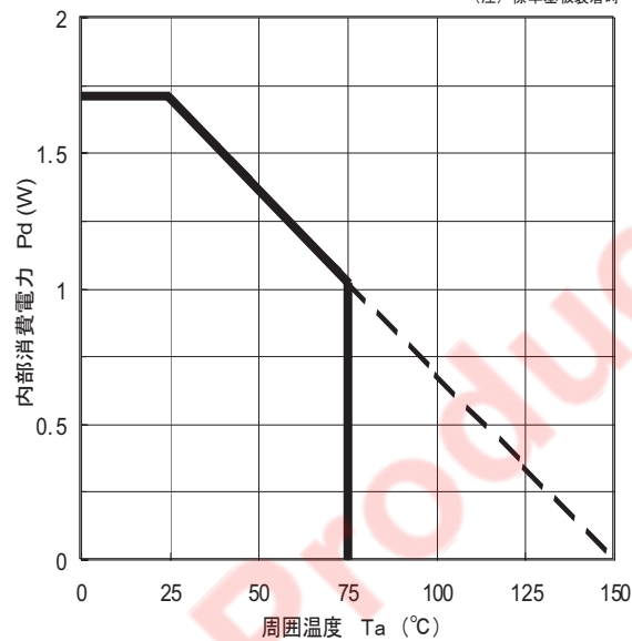
熱低減曲線
