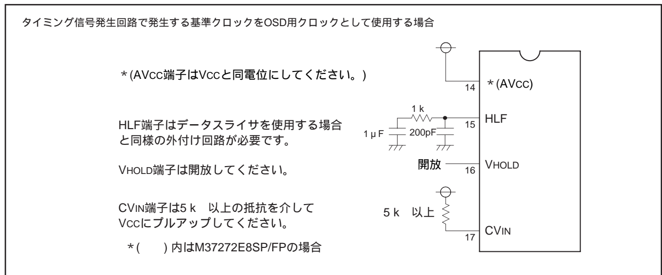
図8.10.3 タイミング信号発生回路 ON の場合の，データスライサ入出力端子の処理方法
