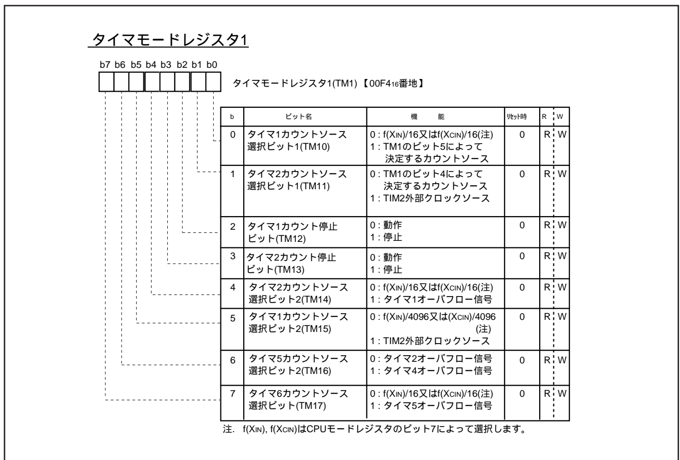
図 8.4.1 タイマモードレジスタ 1
