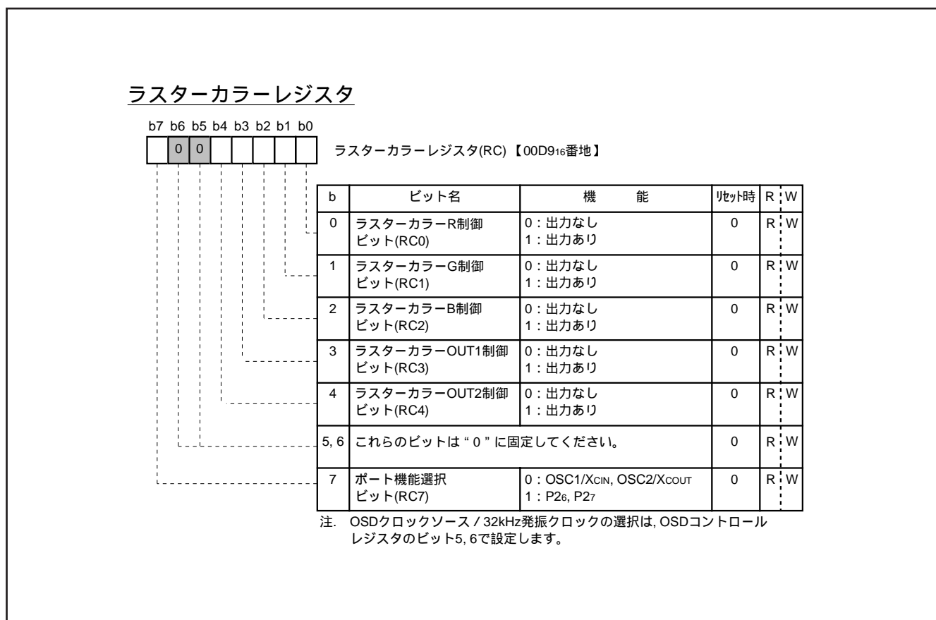
図8.11.29 ラスターカラーレジスタ
