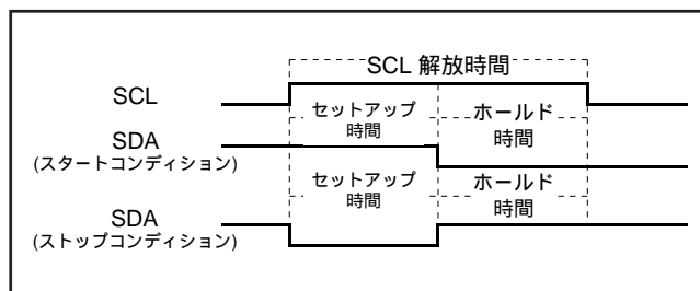
図 8.6.11 スタートコンディション、ストップコンディション検出のタイミング図
