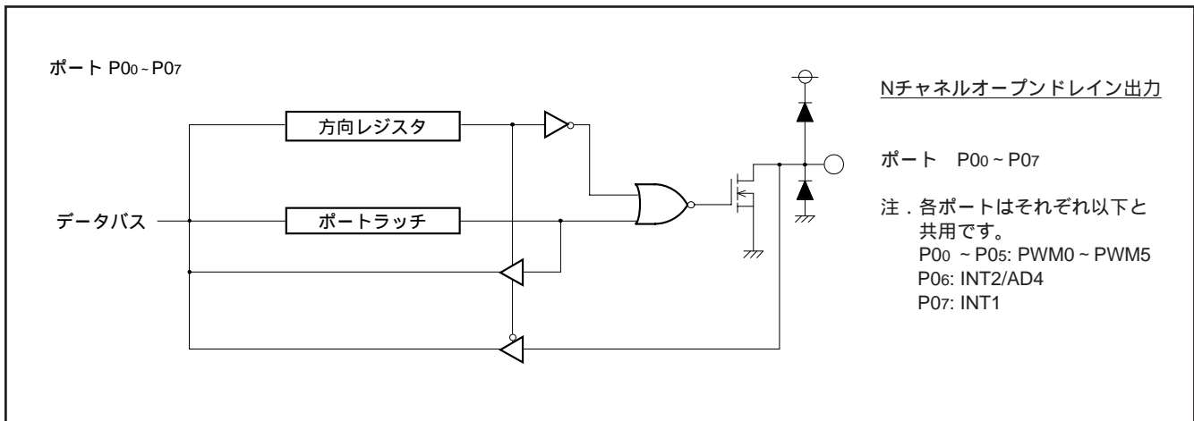
図7.1 入出力端子のブロック図(1)
