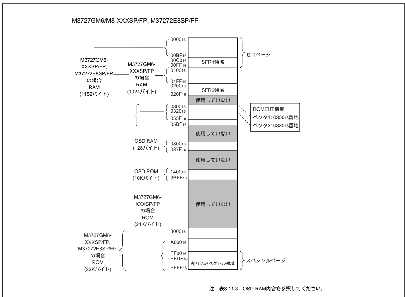
図 8.2.1 メモリ配置図 ( M3727GM6/M8-XXXSP/FP, M37272E8SP/FP )
