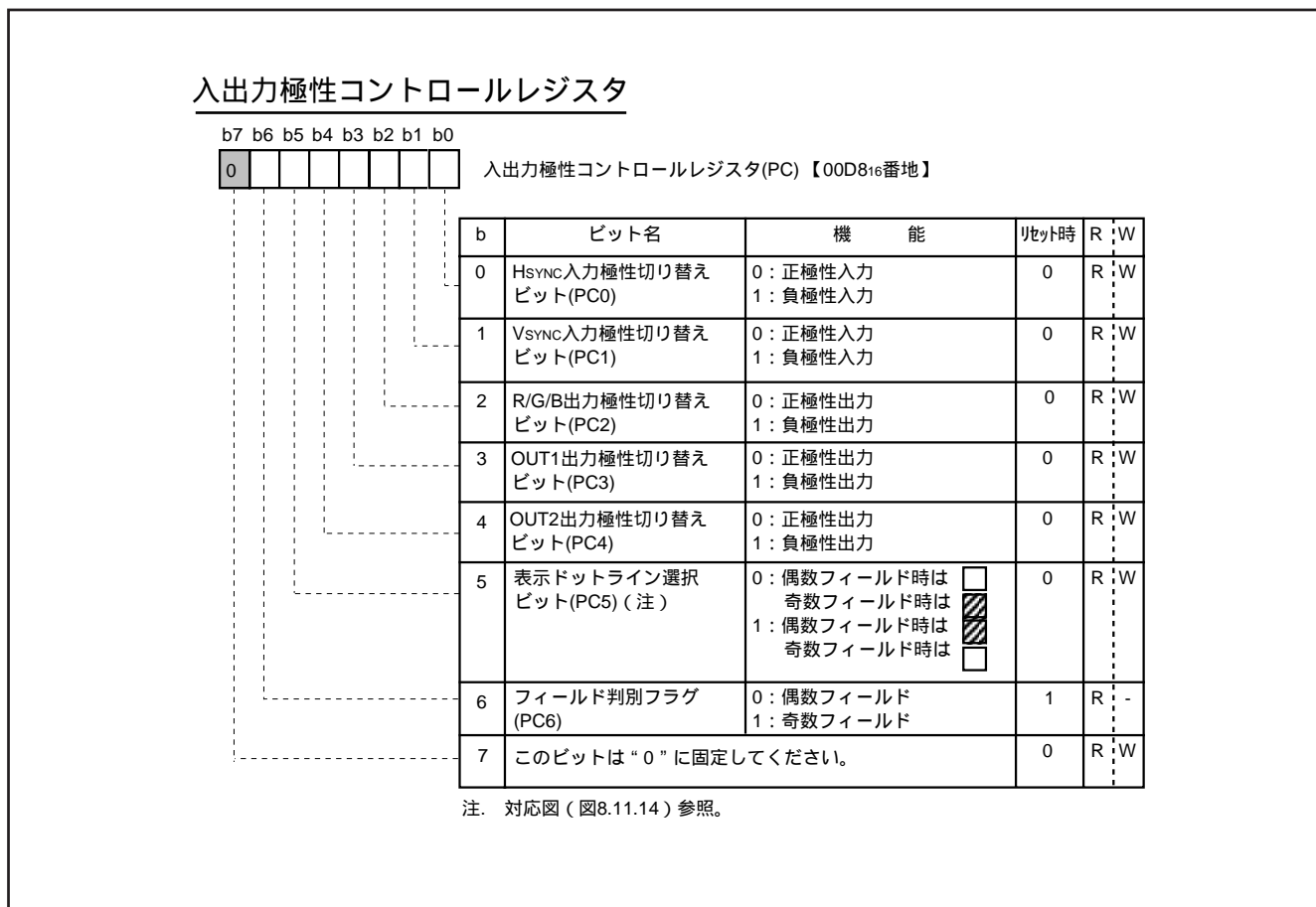
図8.11.13 入出力極性コントロールレジスタ
