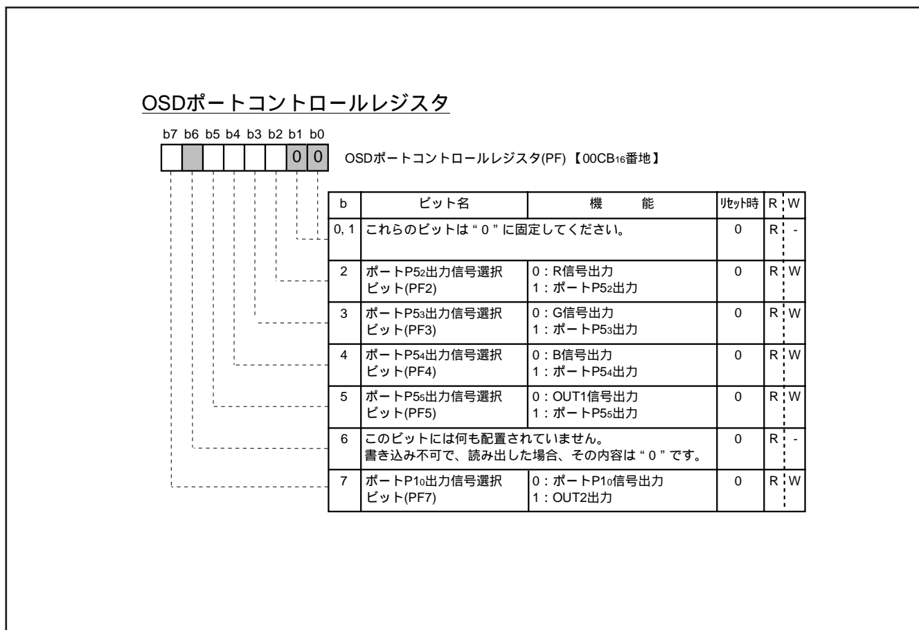
図 8.11.28 OSD ポートコントロールレジスタ
