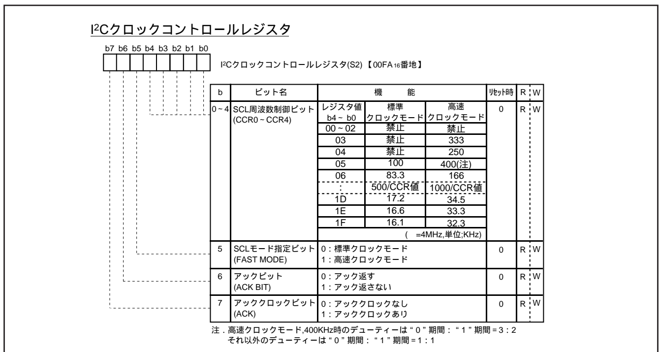
図 8.6.4 I 2 C クロックコントロールレジスタ
