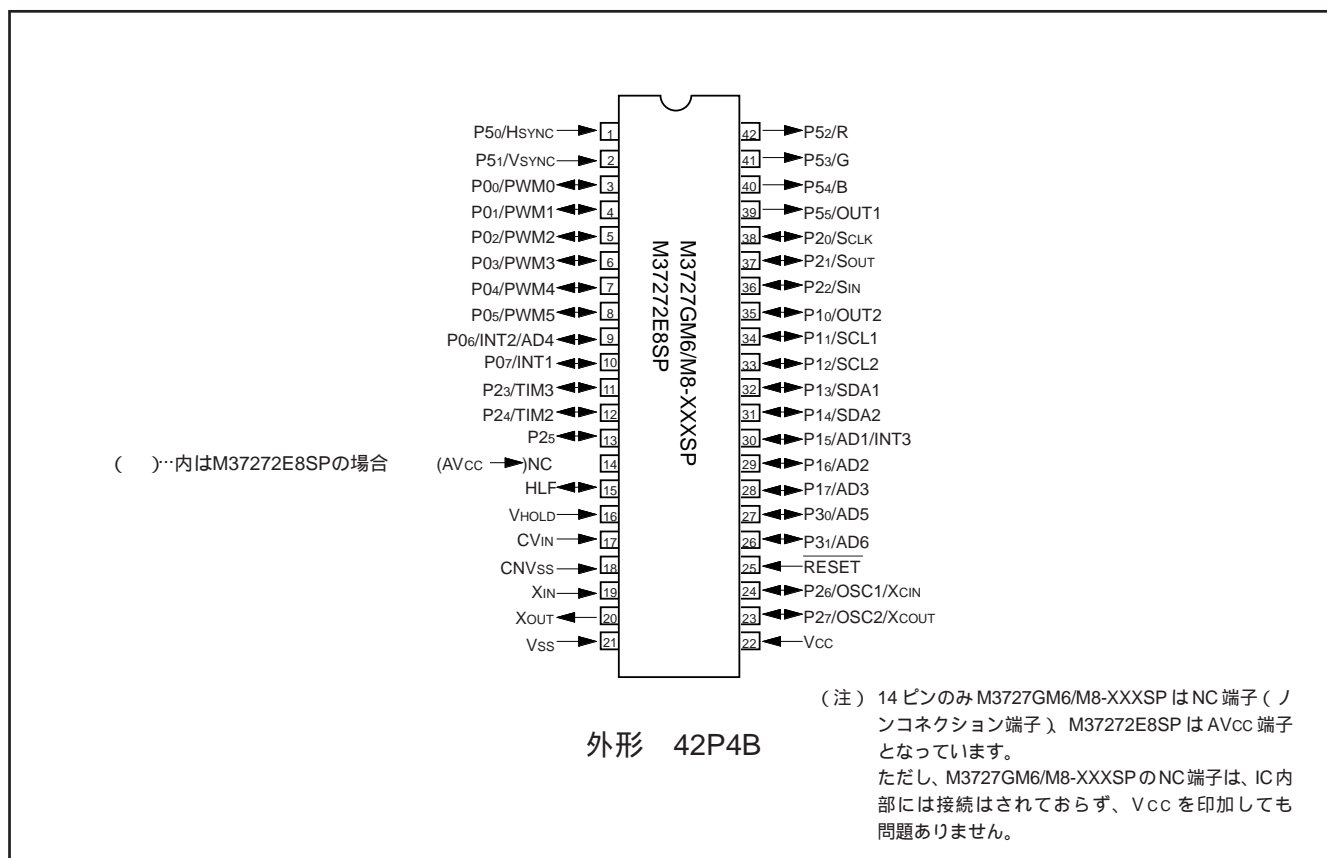
図 4.1 ピン接続図 (1)(上面図)
