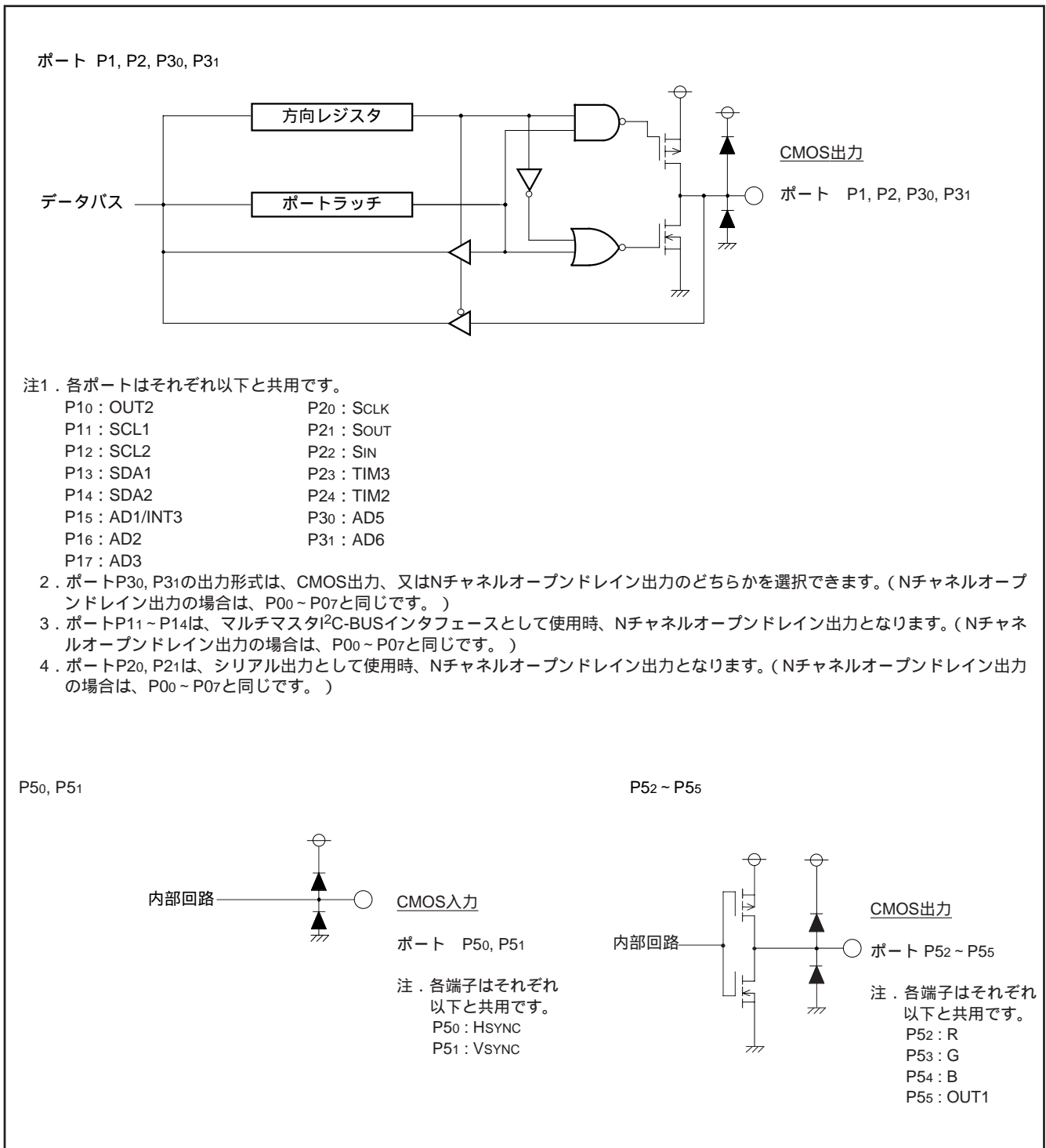
図 7.2 入出力端子のブロック図 (2)
