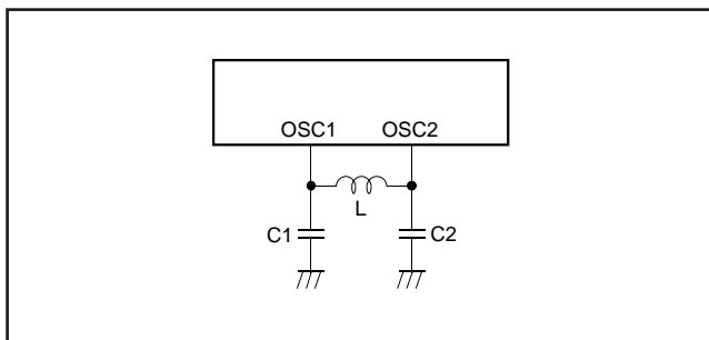
図 8.15.1 OSD用発振回路例
