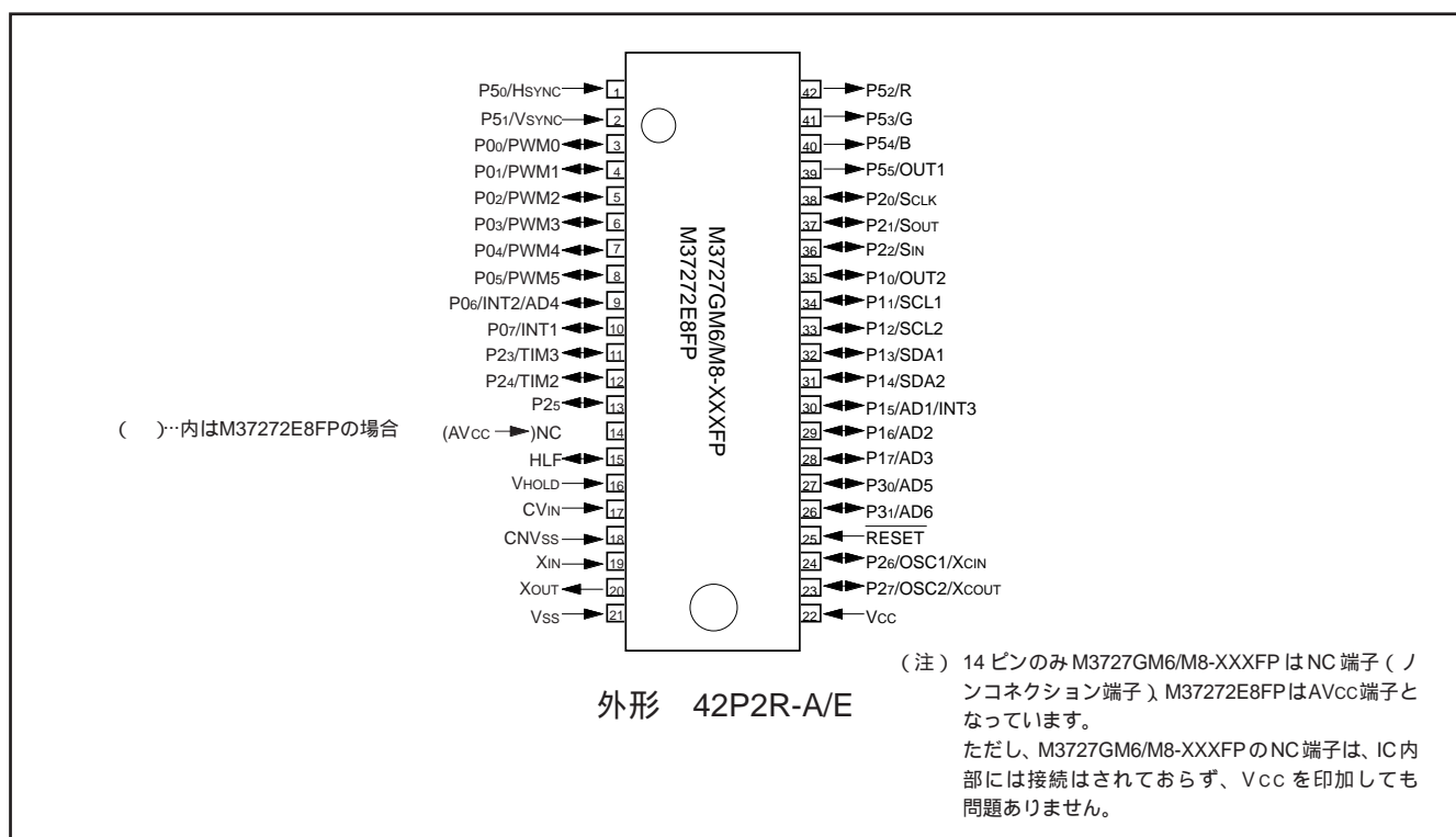
図 4.2 ピン接続図 (2)(上面図)
