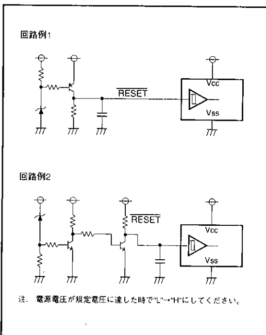
図64. オートクリア回路例
