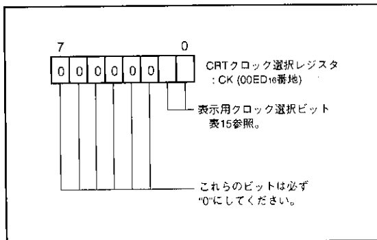
図52. CRTクロック選択レジスタのビット構成
