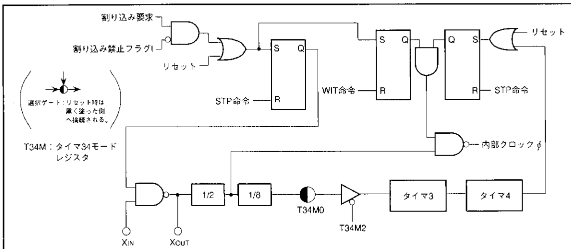
図62. クロック発生回路ブロック図
