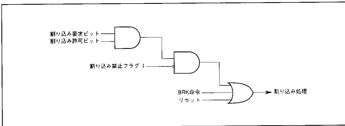
図6. 割り込み制御図
