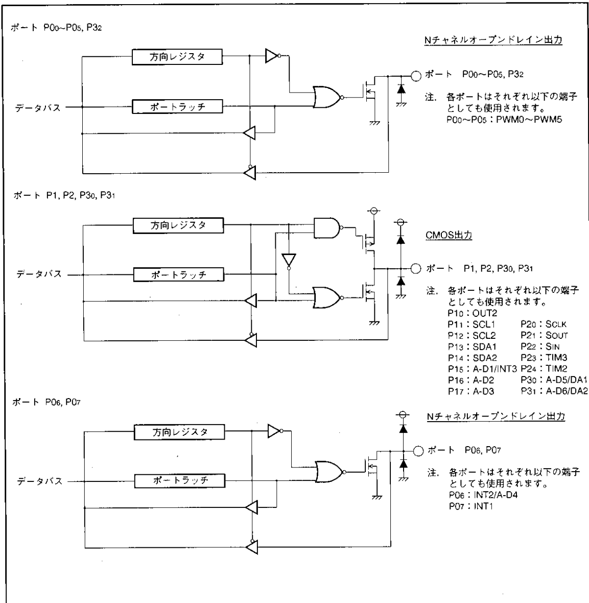
図5B. 入出力端子のブロック図 (1)
