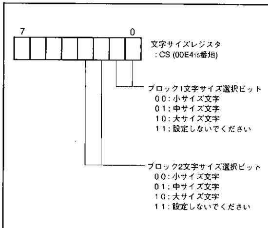
図42. 文字サイズレジスタのビット構成
