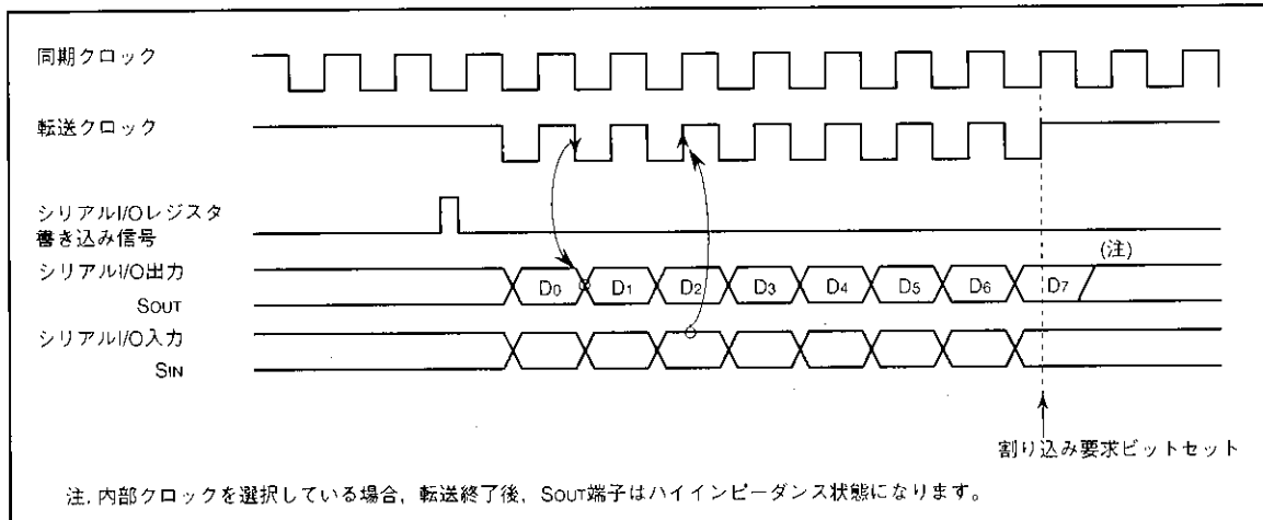
図12. シリアルI/Oタイミング
