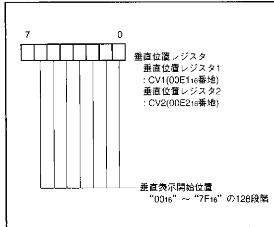
図40. 垂直位置レジスタのビット構成
