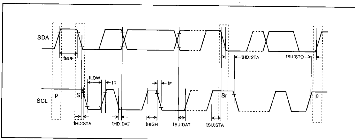
図66. マルチマスタ 2 C-BUSのタイミング定義図
