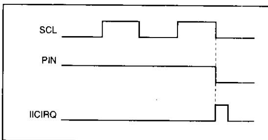
図20. 割り込み要求信号の発生タイミング
