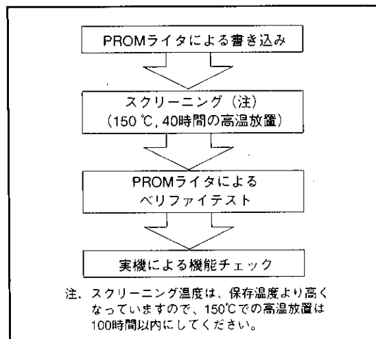
図65. ワンタイムPROM版書き込みとテスト
