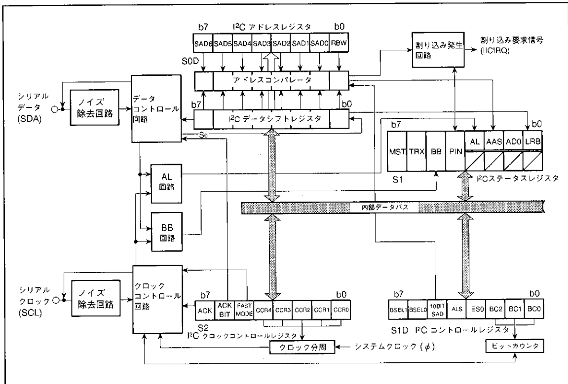
図14. マルチマスタI 2 C-BUSインタフェースのブロック図
