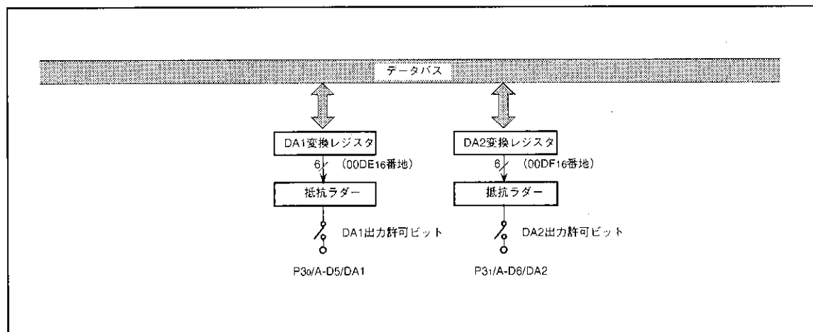
図34. D-A変換器ブロック図
