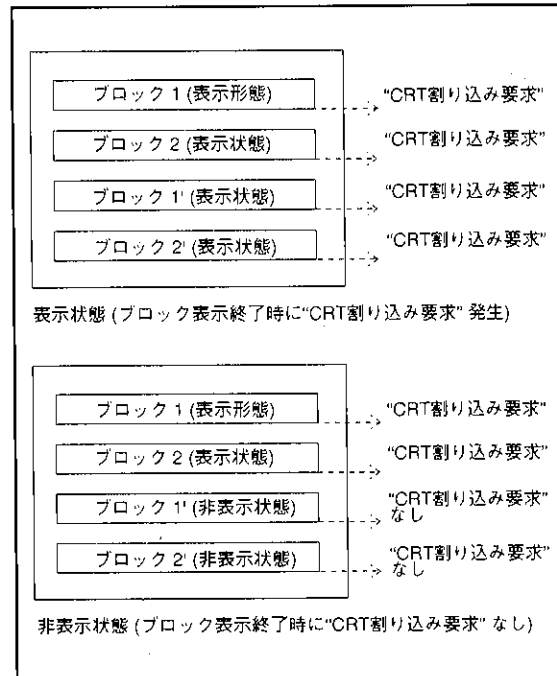
図49. CRT割り込みのタイミング
