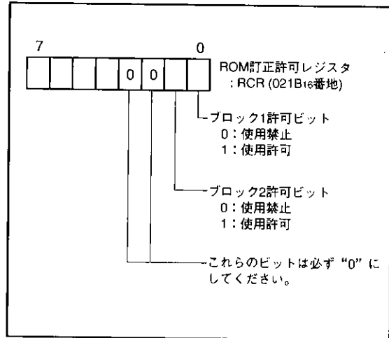
図54. ROM訂正許可レジスタのビット構成
