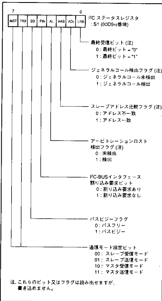
図19. I 2 Cステータスレジスタのビット構成
