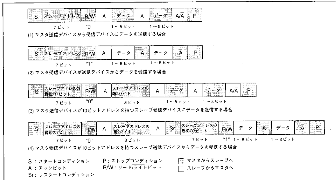
図24. アドレスデータ通信フォーマット
