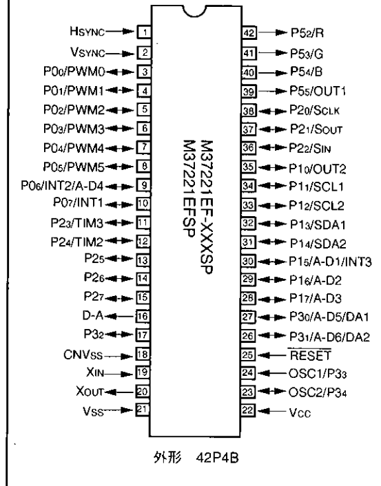
ピン接続図(上面図)
