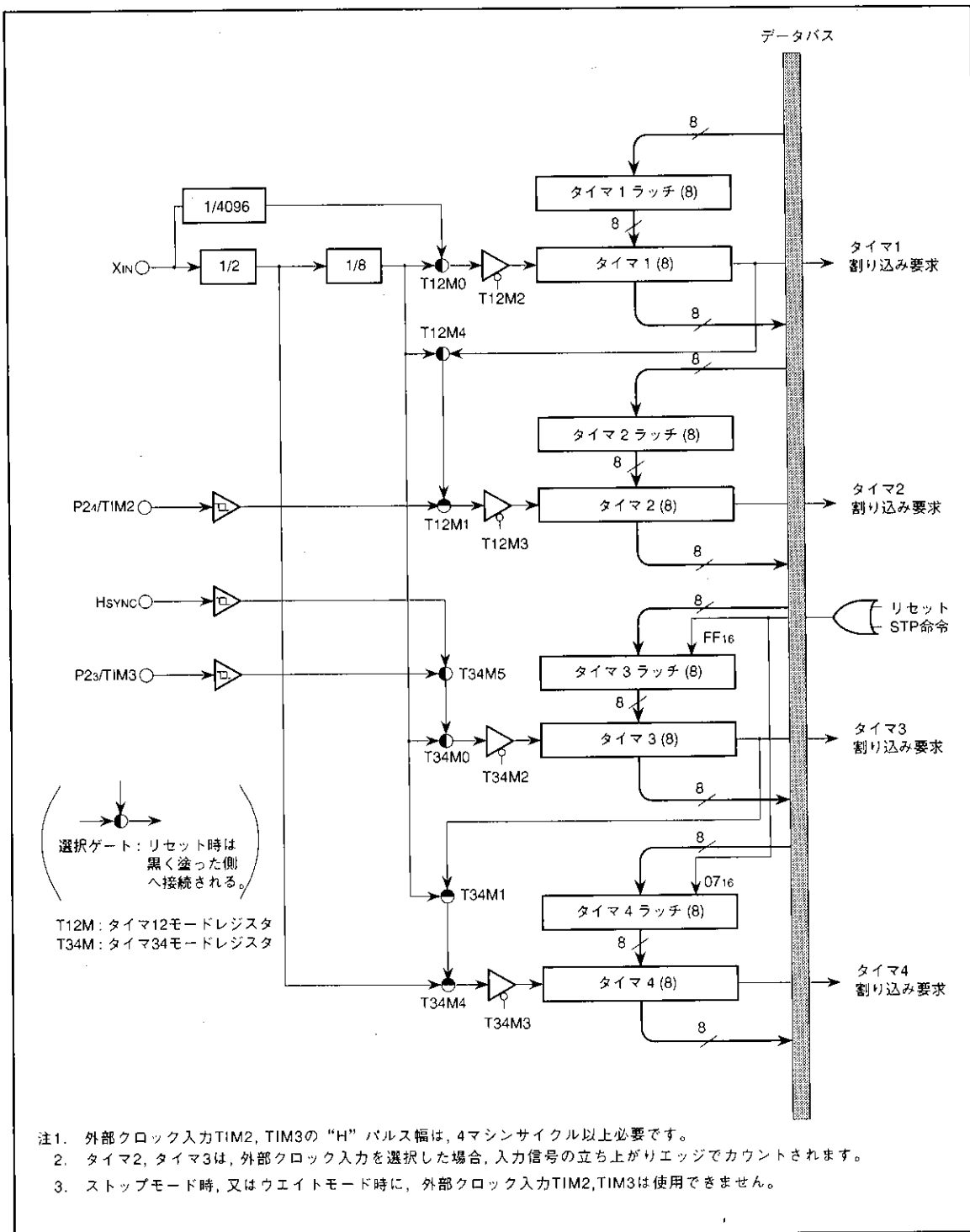
図9. タイマブロック図
