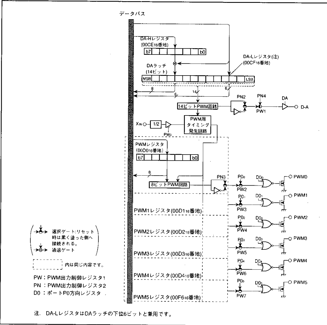
図25. PWM回路ブロック図
