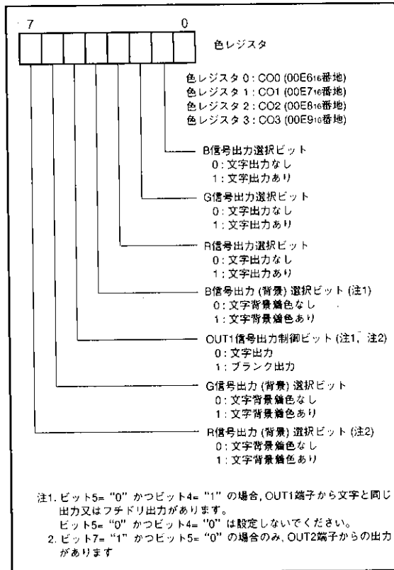
図46. 色レジスタのビット構成
