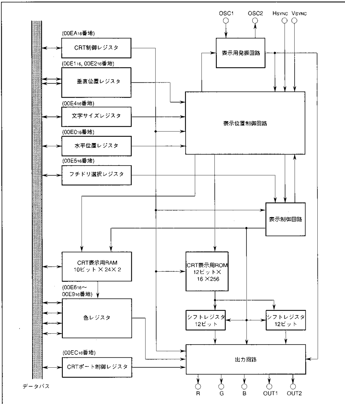
図37. CRT表示制御回路ブロック図
