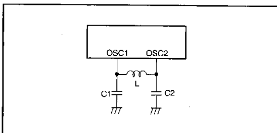
図63. 表示用発振回路例
