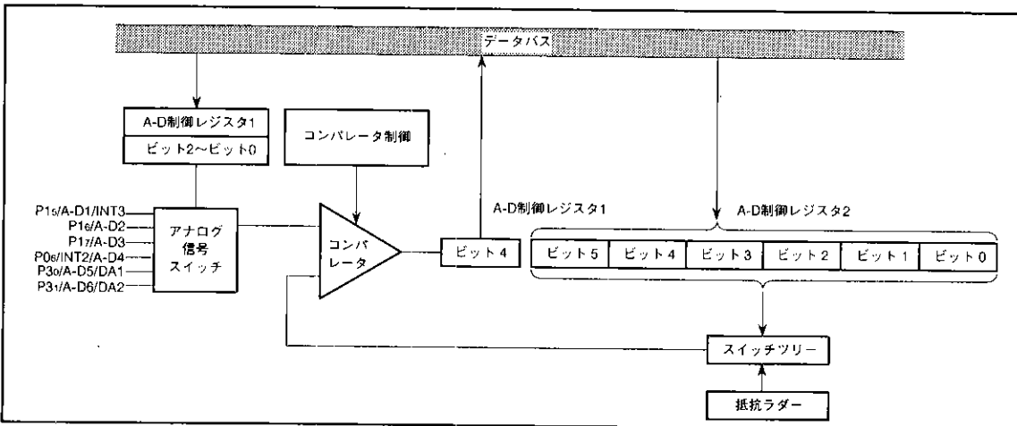
図31. A-D比較器ブロック図
