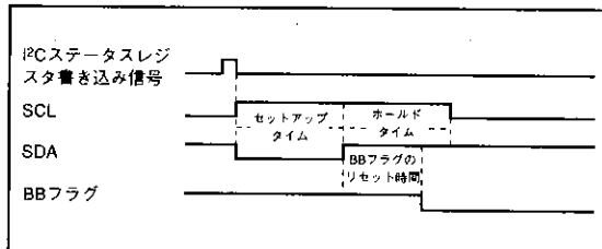
図22. ストップコンディション発生タイミング図
