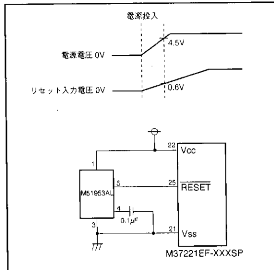
図55. リセット回路例
