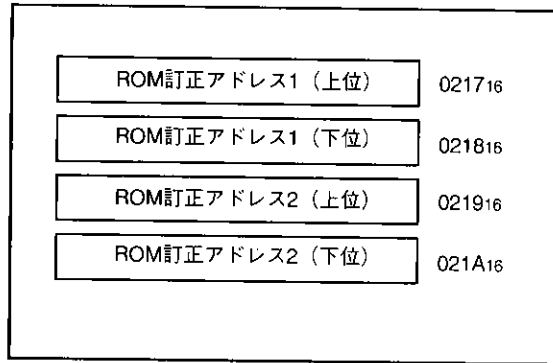
図53. ROM訂正アドレス
