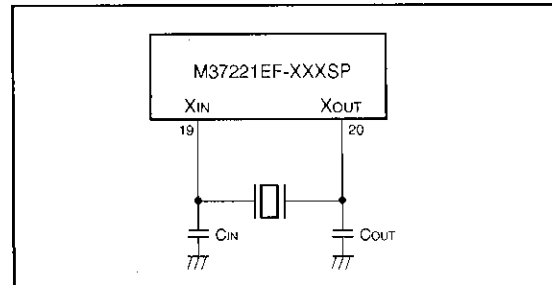
図60. セラミック共振子外付け回路例
