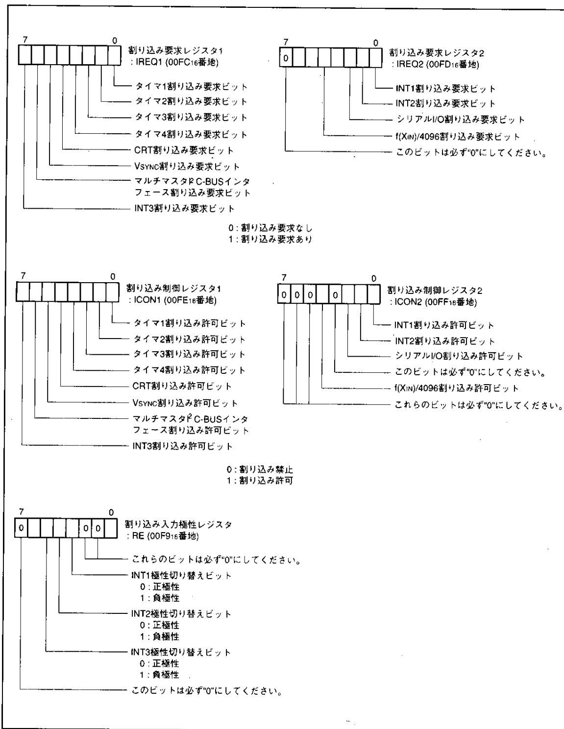
図7. 割り込み関係レジスタのビット構成
