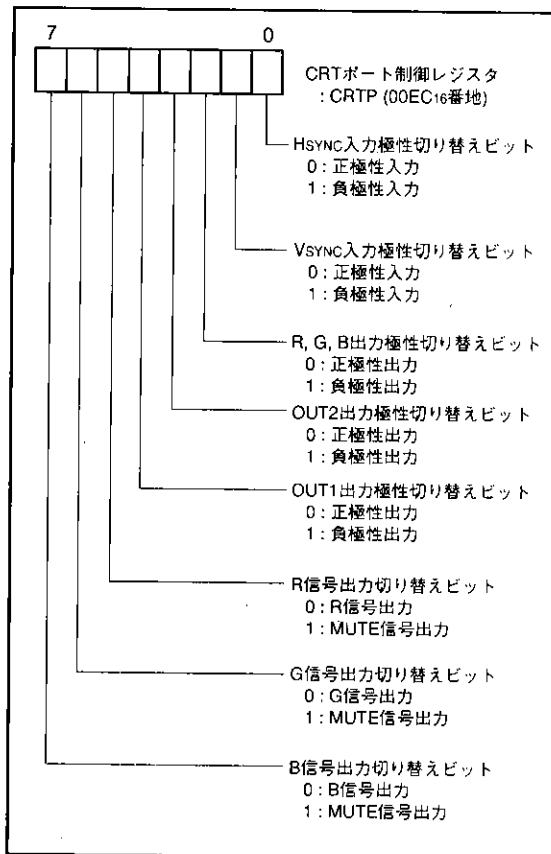
図50. CRTポート制御レジスタのビット構成
