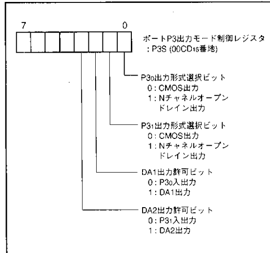
図33. ポートP3出力モードレジスタのビット構成
