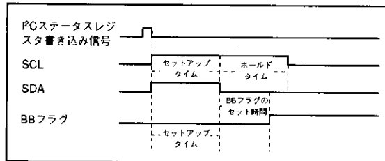
図21. スタートコンディション発生タイミング図
