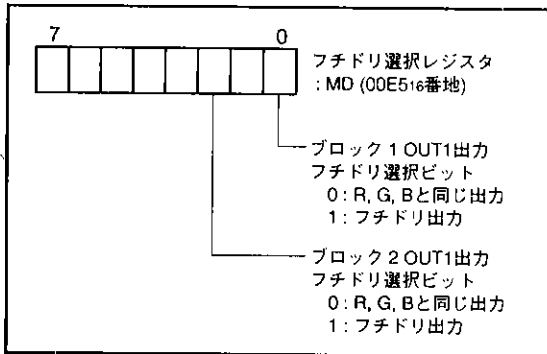
図47. フチドリ選択レジスタのビット構成
