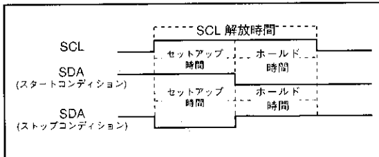
図23. スタートコンディション、ストップコンディション検出のタイミング図
