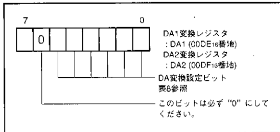
図32. DA変換レジスタのビット構成
