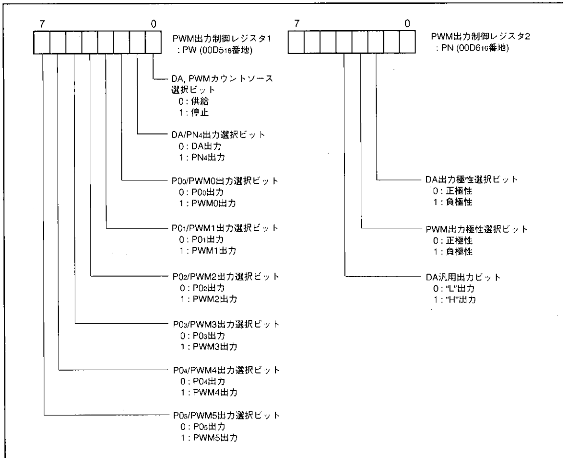
図28. PWM関係レジスタのビット構成
