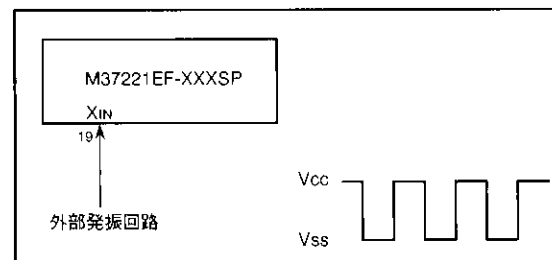
図61. 外部クロック入力回路例
