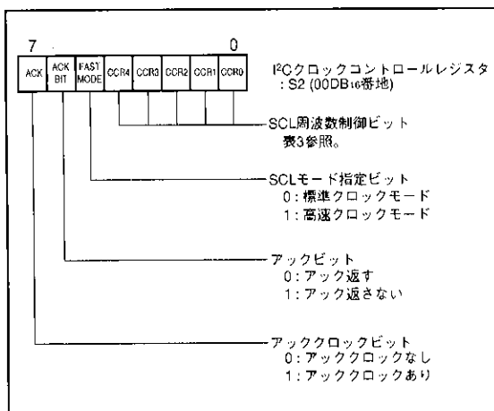
図16. I 2 Cクロックコントロールレジスタのビット構成
