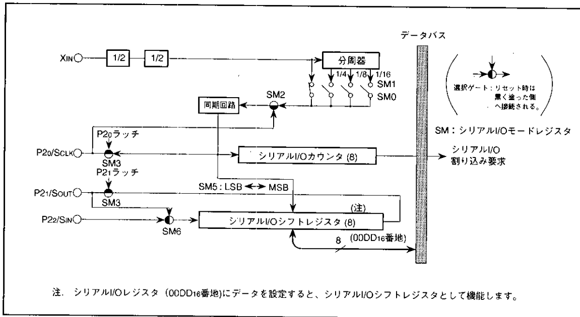
図10. シリアルI/Oのブロック図
