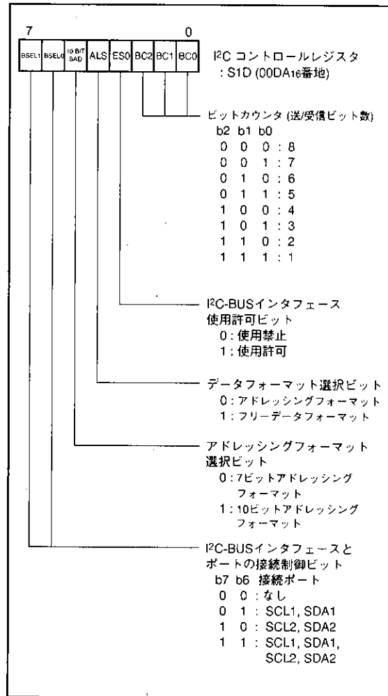
図18. I 2 Cコントロールレジスタのビット構成
