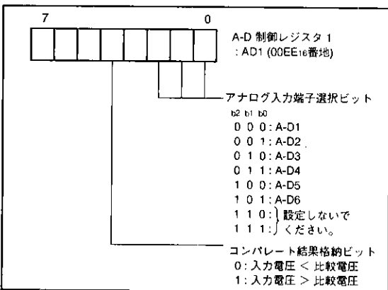
図29. A-D制御レジスタ1のビット構成
