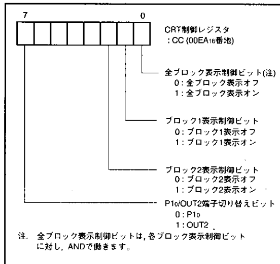
図36. CRT制御レジスタのビット構成
