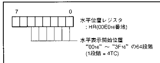
図41. 水平位置レジスタのビット構成
