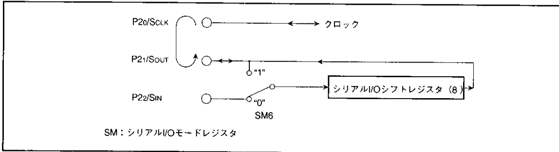
図13. シリアルI/O共用送受信モード時の信号
