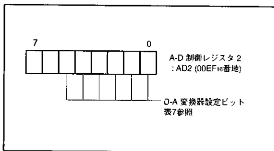
図30. A-D制御レジスタ2のビット構成
