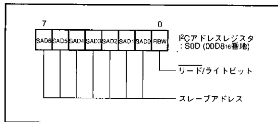
図15. I 2 Cアドレスレジスタのビット構成
