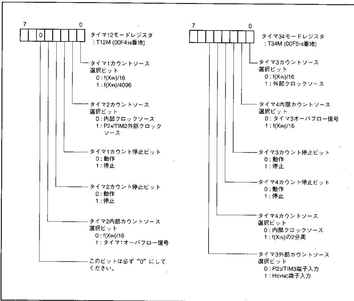
図8. タイマ関係レジスタのビット構成
