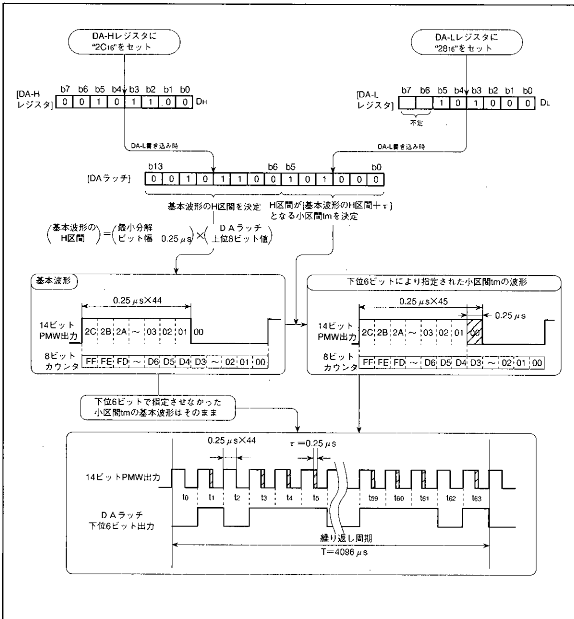
図27. 14ビットPWMタイミング図 ( f(XIN) = 8MHz )
