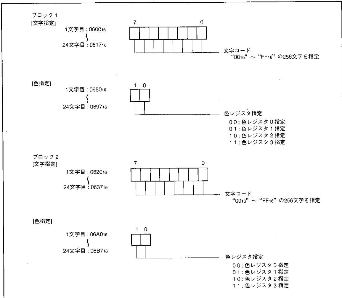
図45. CRT表示用RAMのビット構成
