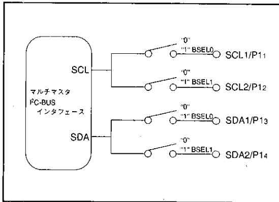
図17. BSEL0, BSEL1による接続ポート制御
