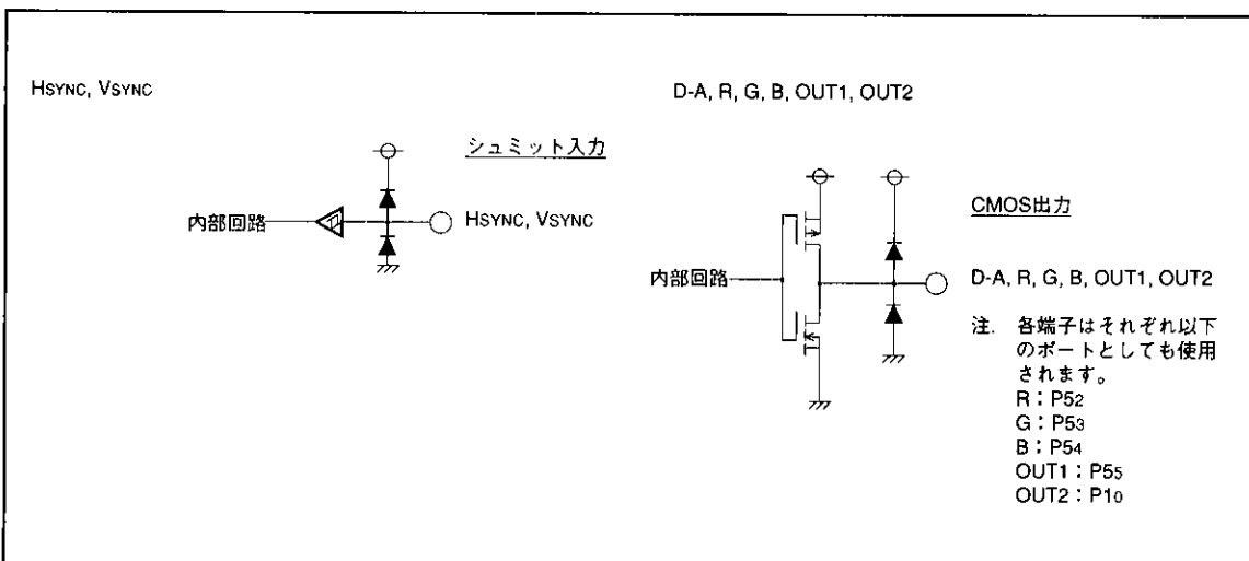
図59. 入出力端子のブロック図 (2)
