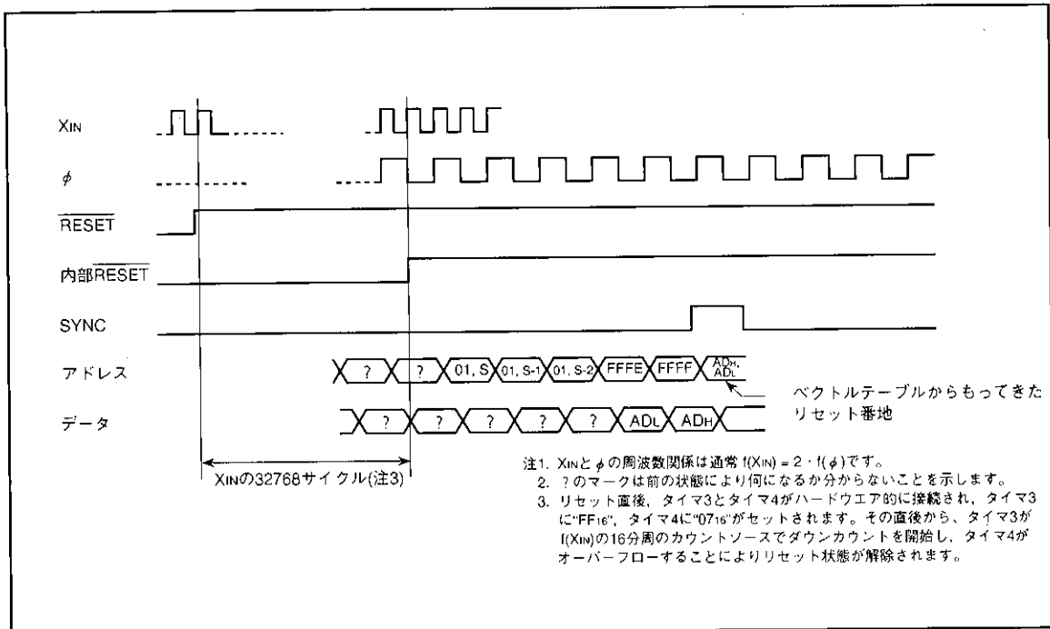
図56. リセット時のタイミング図
