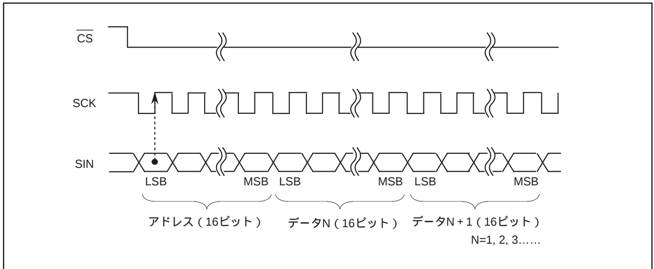
図11 . データ入力タイミング
