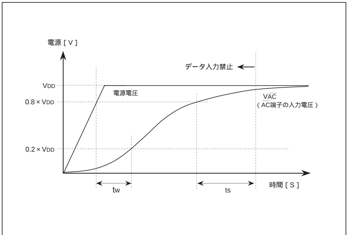
図17. \overline{AC} 端子への電源投入タイミング
