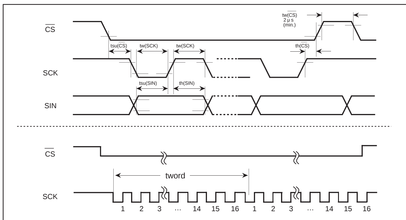
図16．シリアル入力タイミング条件
