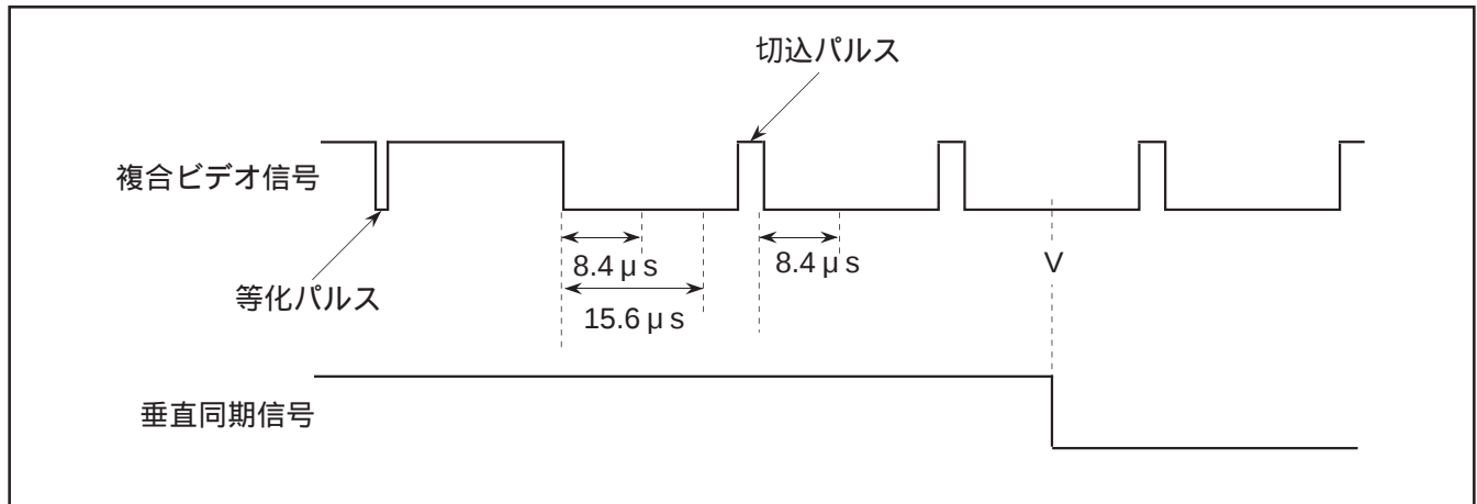
図5．複合ビデオ信号から同期分離の仕方
