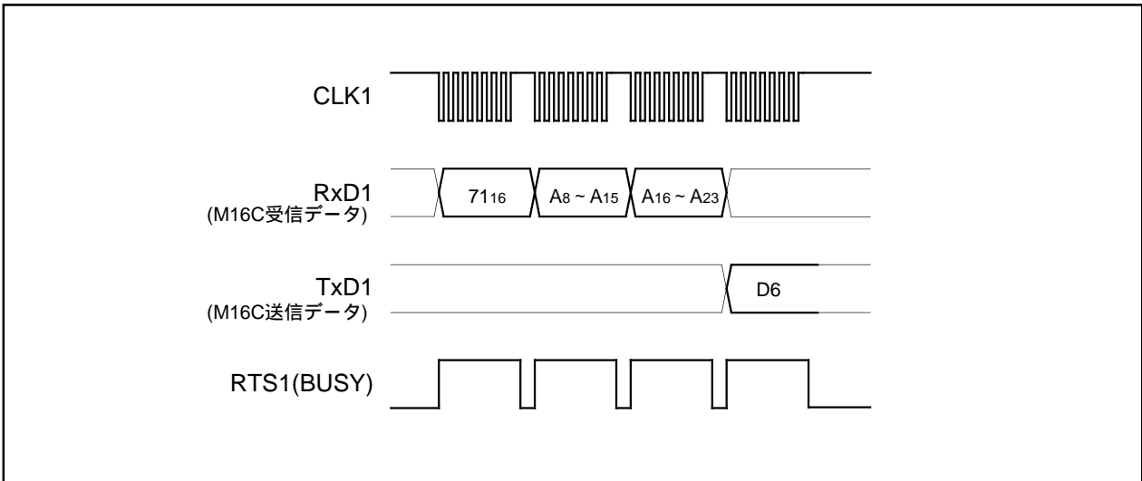
図1.25.9. リードロックビットステータスコマンド時のタイミング
