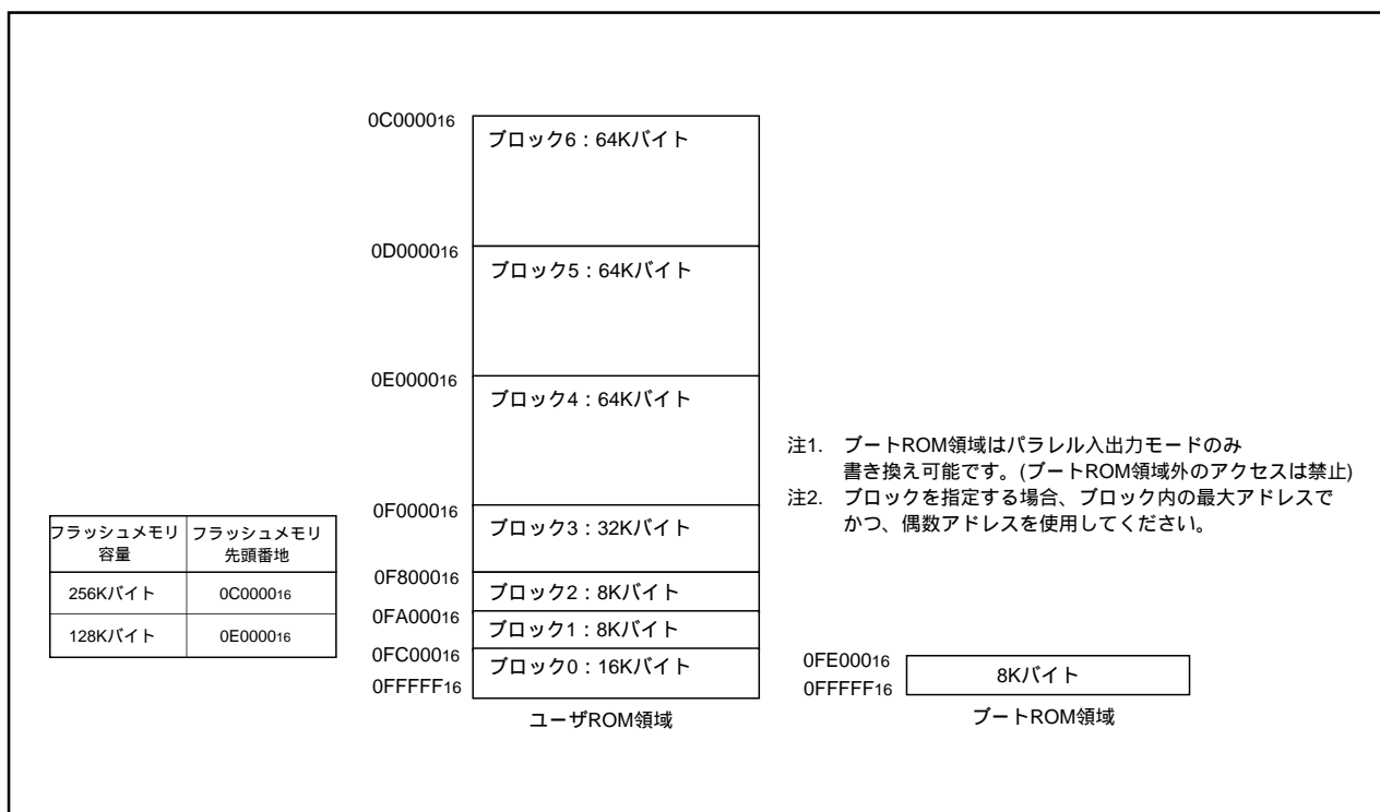
図1.21.1. 内蔵フラッシュメモリのブロック図
