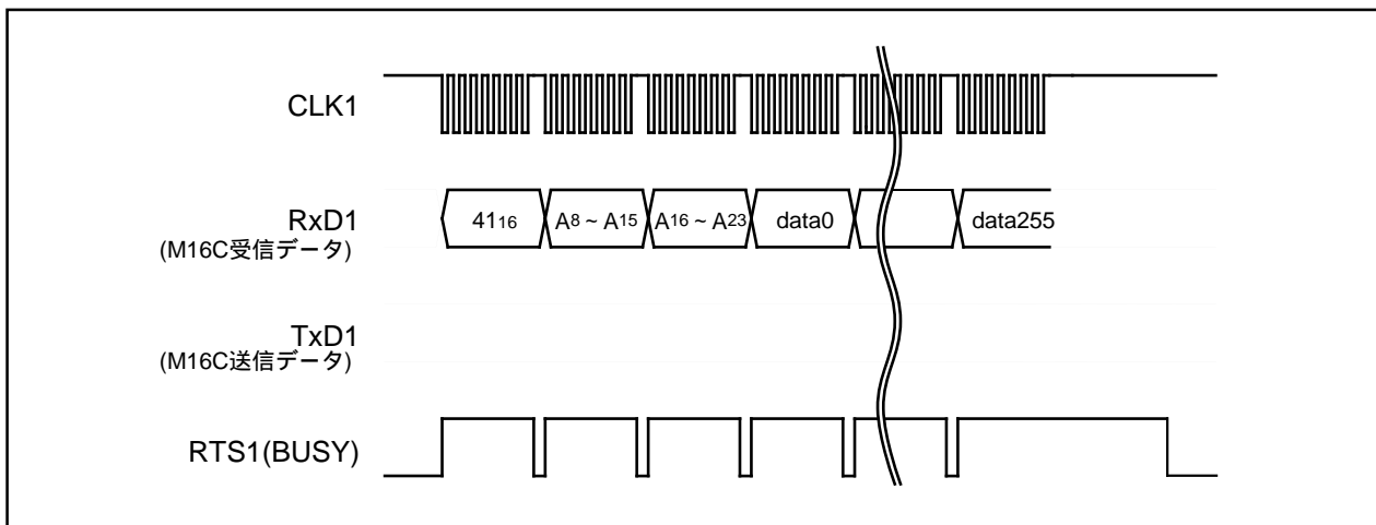
図1.25.5. ページプログラムコマンド時のタイミング
