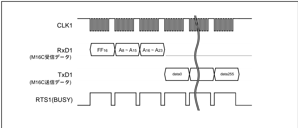
図1.25.2. ページリードコマンド時のタイミング
