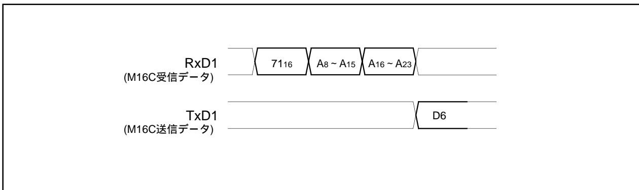
図1.25.29. リードロックビットステータスコマンド時のタイミング
