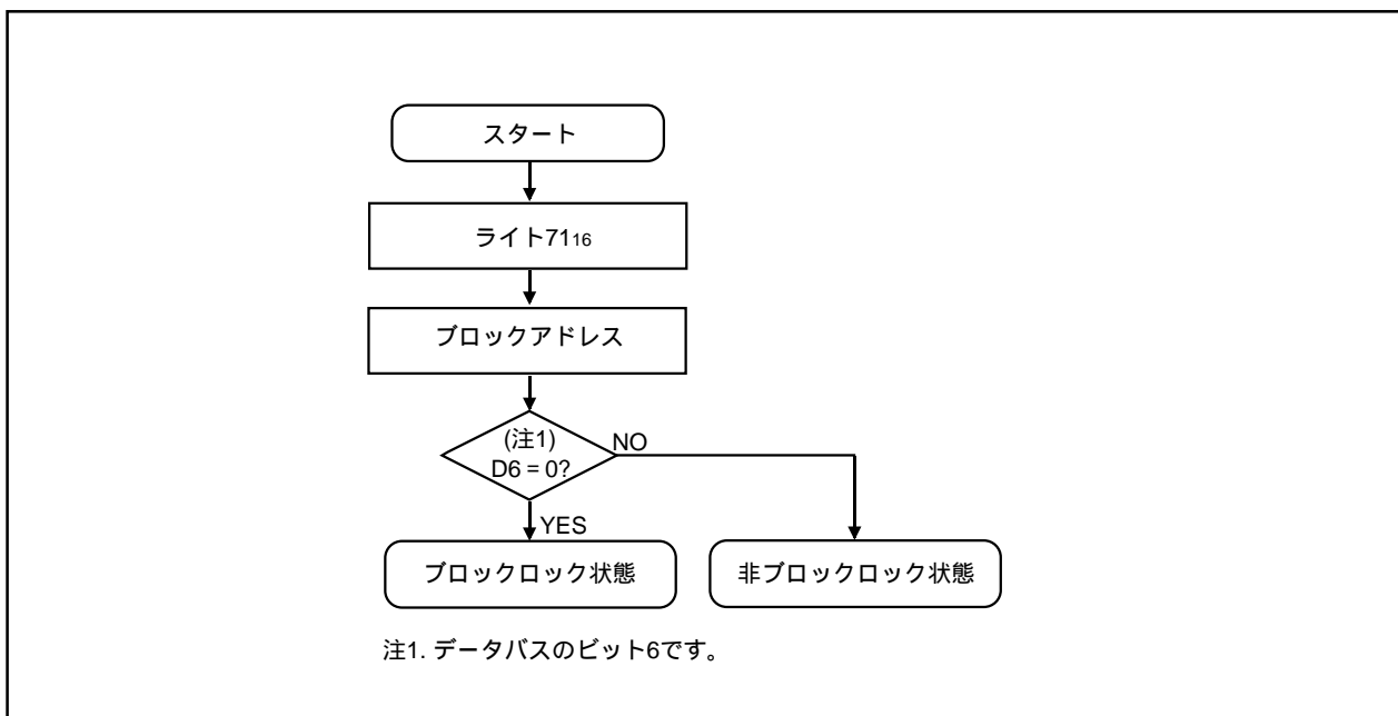
図1.22.7. リードロックビットステータスフローチャート
