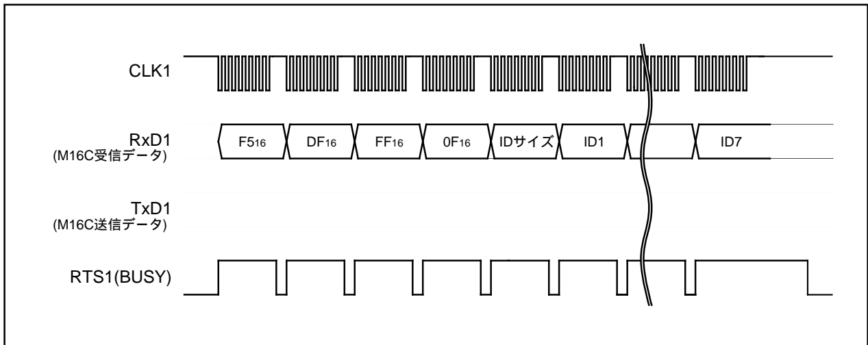
図1.25.15. IDチェック機能のタイミング
