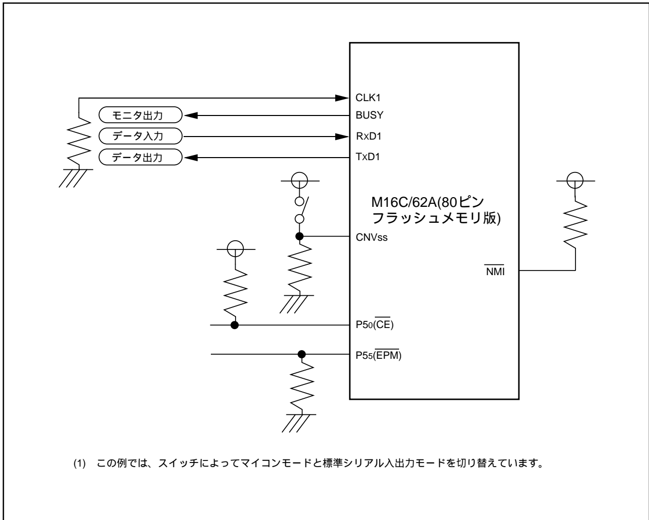
図1.25.42. 標準シリアル入出力モード2時の応用回路例
