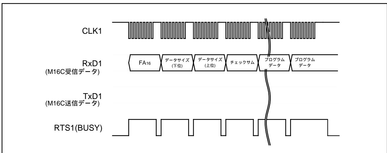
図1.25.12. ダウンロード機能のタイミング
