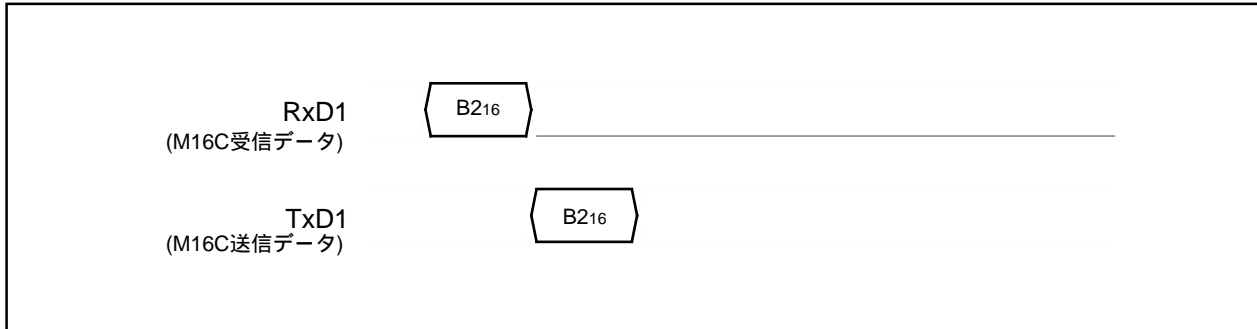
図1.25.40. ボーレート38400のタイミング
