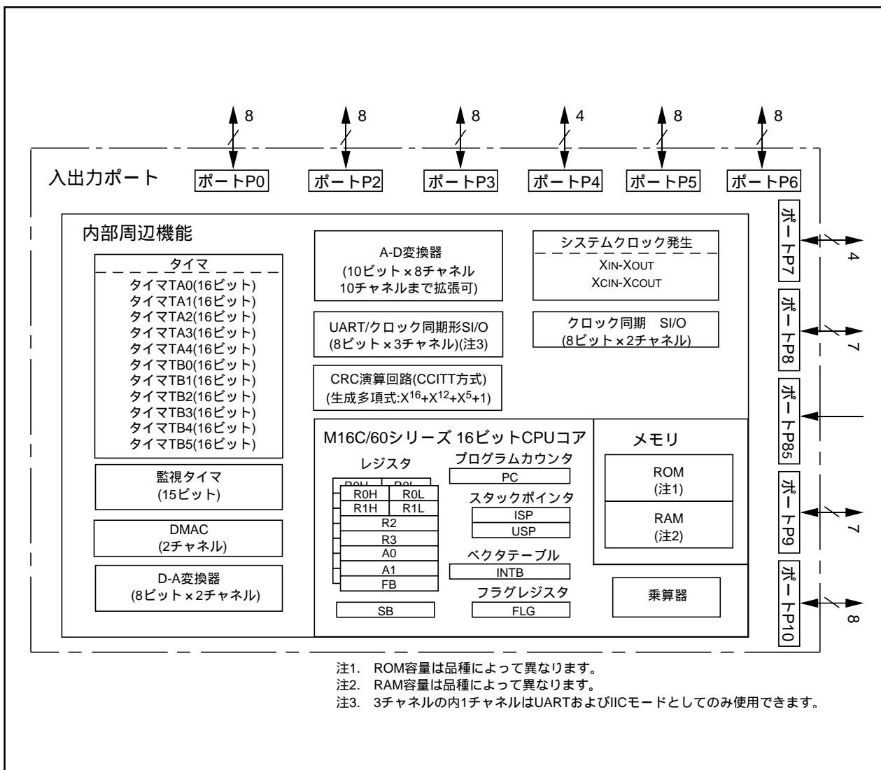
図1.1.2. M16C/62A(80ピン版)グループのブロック図
