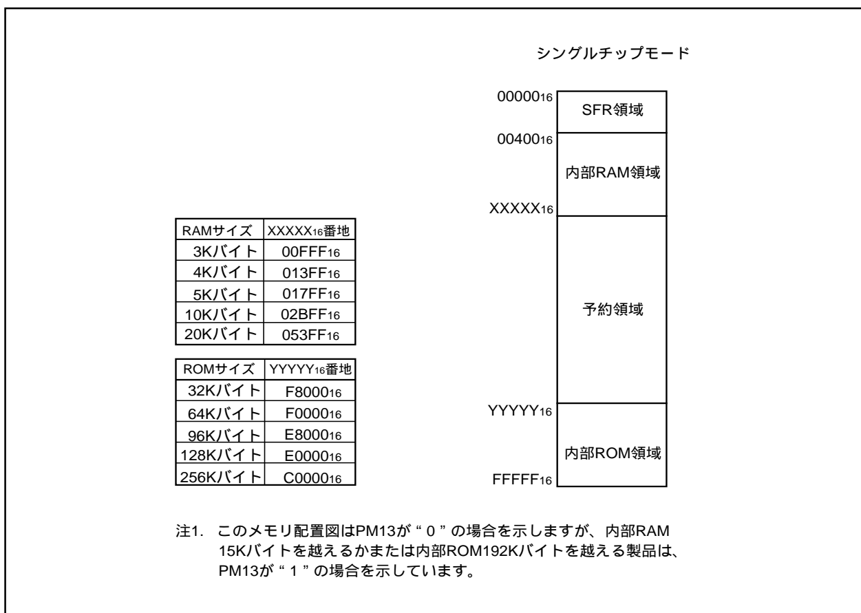
図1.8.2. メモリ配置
