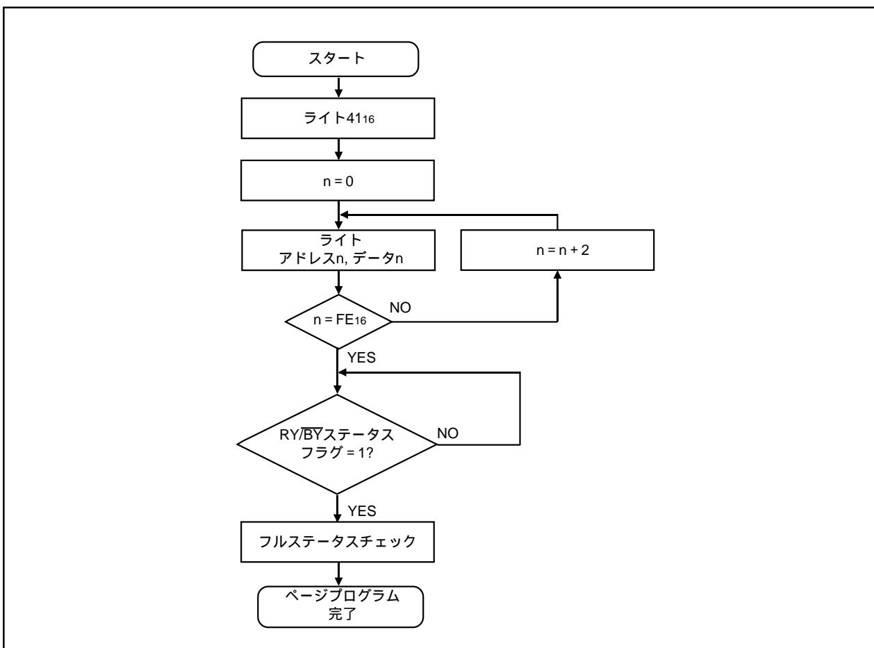
図1.22.4. ページプログラムフローチャート
