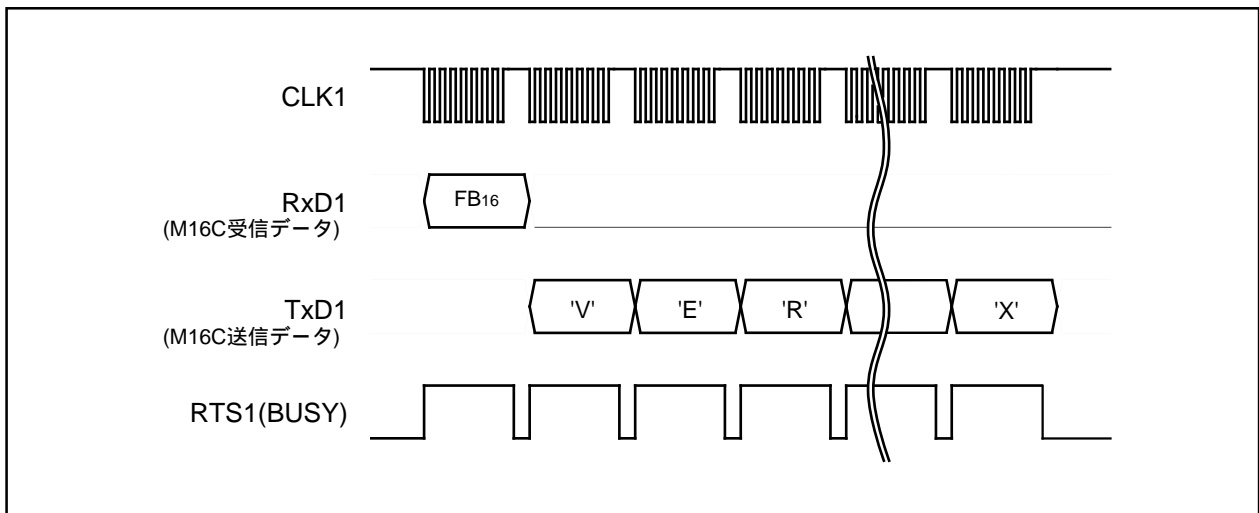
図1.25.13. バージョン情報出力機能のタイミング
