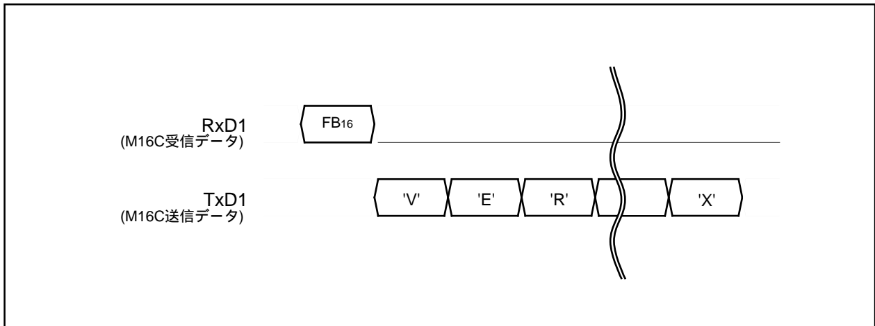
図1.25.33. バージョン情報出力機能のタイミング
