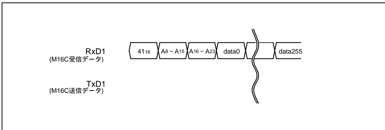
図1.25.25. ページプログラムコマンド時のタイミング
