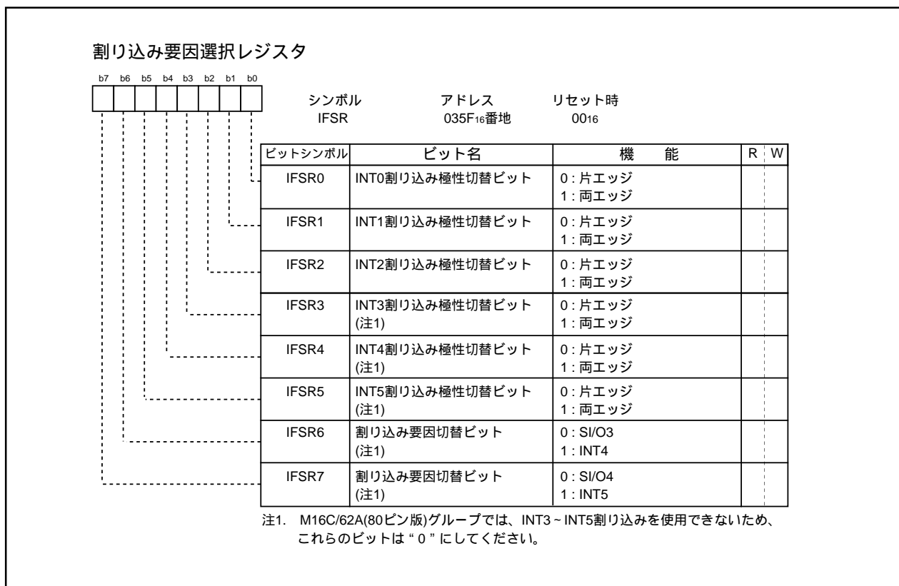
図1.10.10. 割り込み要因選択レジスタの構成
