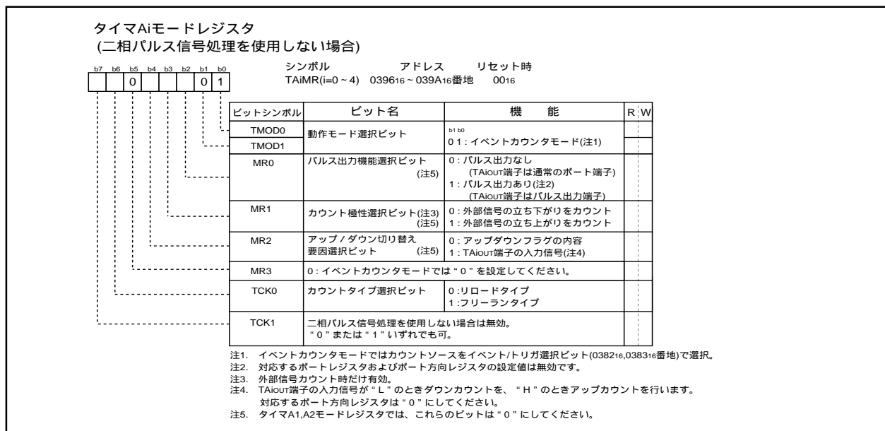
図1.13.8. イベントカウンタモード時のタイマAiモードレジスタの構成
