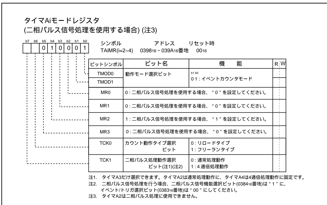
図1.13.9. イベントカウンタモード時のタイマAiモードレジスタの構成
