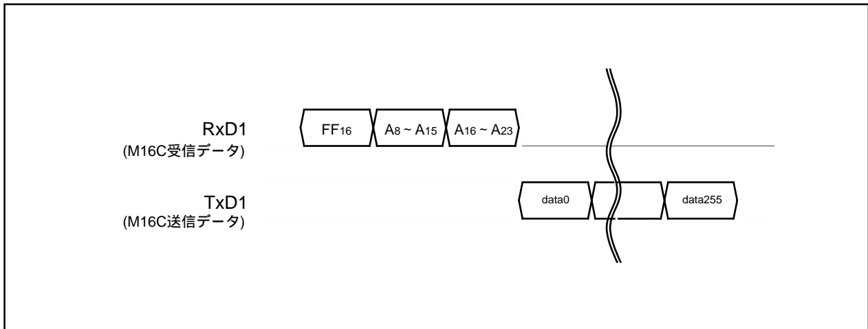
図1.25.22. ページリードコマンド時のタイミング
