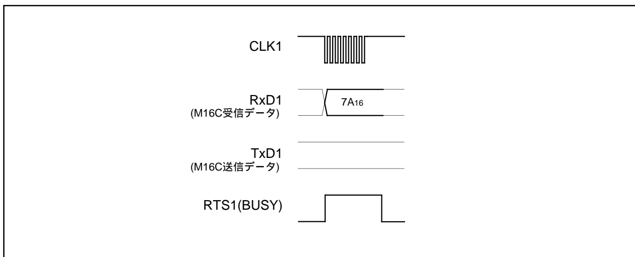
図1.25.10. ロックビット有効コマンド時のタイミング
