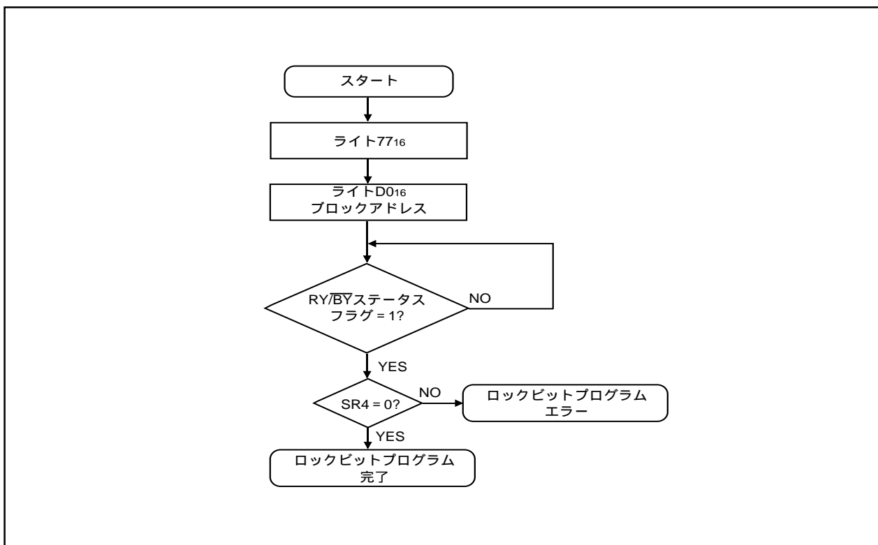
図1.22.6. ロックビットプログラムフローチャート
