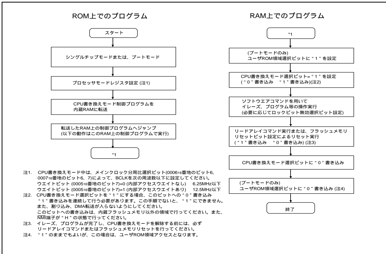
図1.22.2. CPU書き換えモードの設定/解除フローチャート
