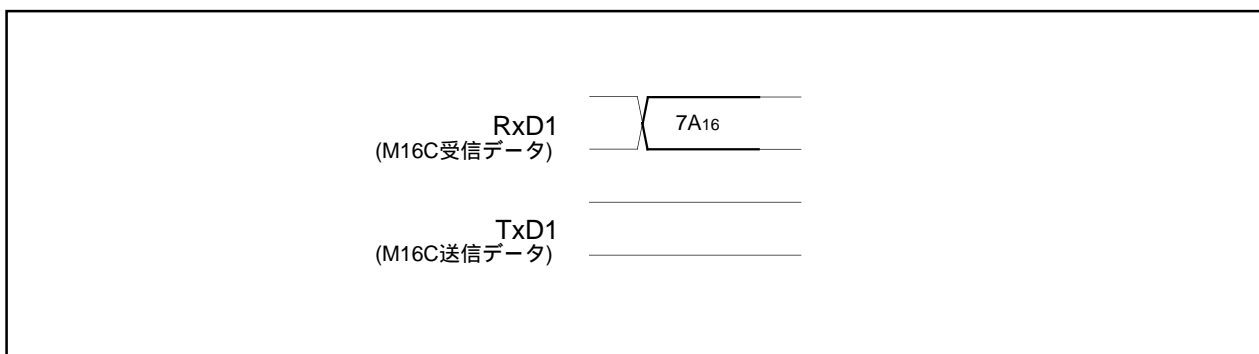
図1.25.30. ロックビット有効コマンド時のタイミング
