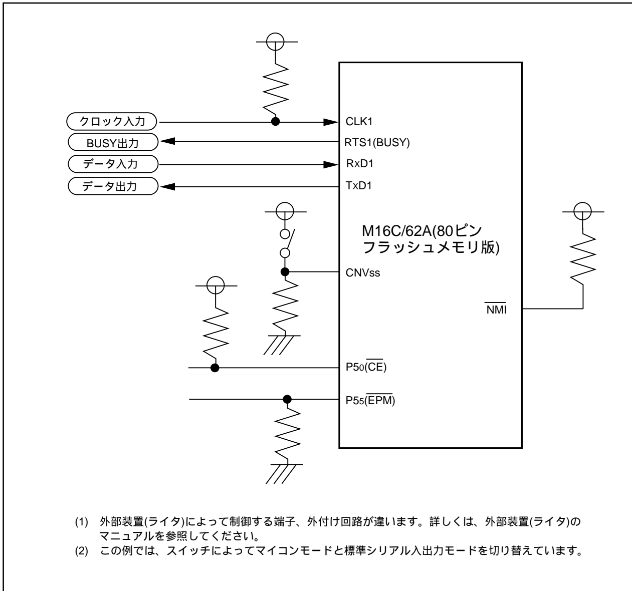
図1.25.20. 標準シリアル入出力モード1時の応用回路例
