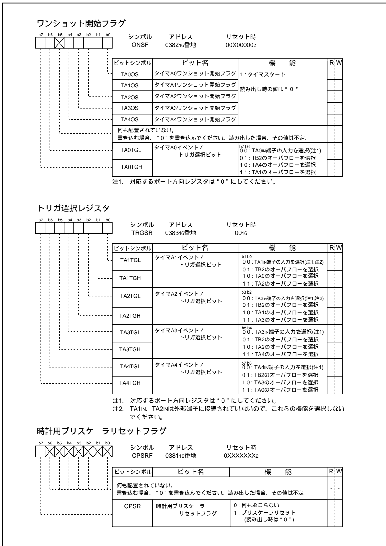
図1.13.6. タイマA関連レジスタ(3)
