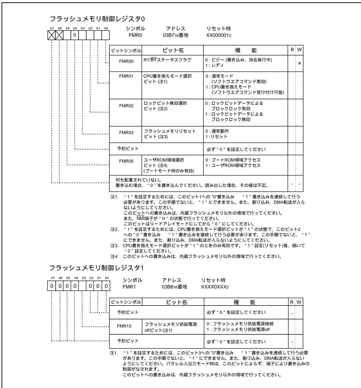
図1.22.1. フラッシュメモリ制御レジスタ0、フラッシュメモリ制御レジスタ1
