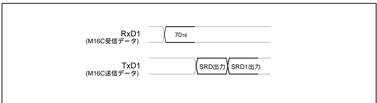
図1.25.23. リードステータスレジスタコマンド時のタイミング
