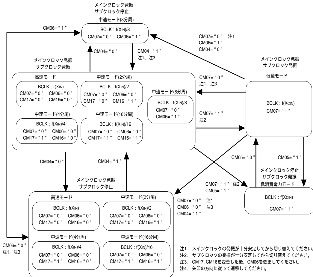
図1.9.5. 状態遷移図
