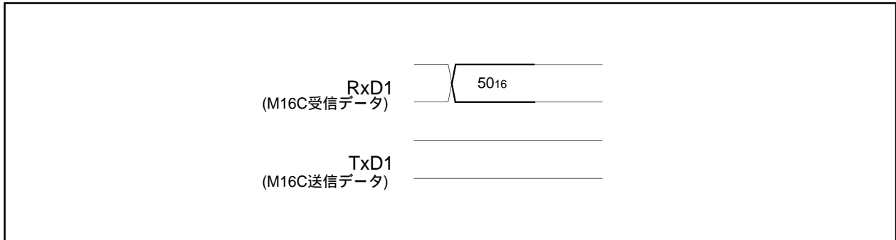
図1.25.24. クリアステータスレジスタコマンド時のタイミング
