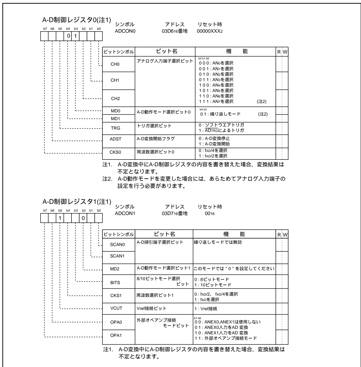
図1.15.5. 繰り返しモード時のA-D制御レジスタ
