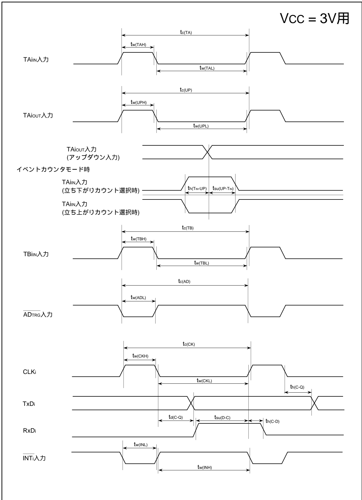
図1.20.2. Vcc=3V用タイミング図
