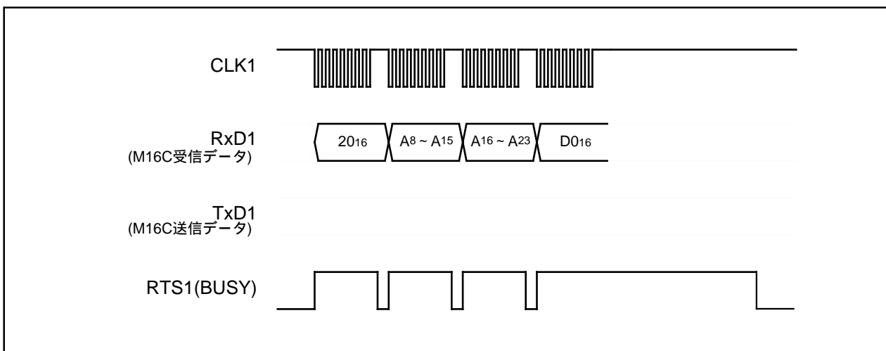
図1.25.6. ブロックイレーズコマンド時のタイミング
