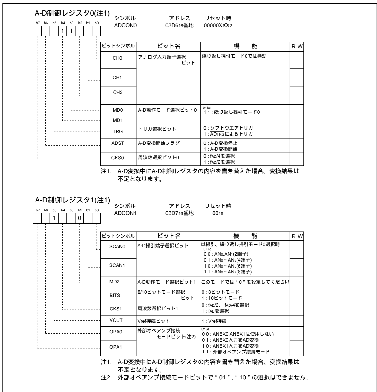
図1.15.7. 繰り返し掃引モード0時のA-D制御レジスタ
