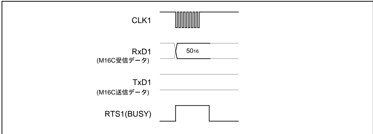
図1.25.4. クリアステータスレジスタコマンド時のタイミング
