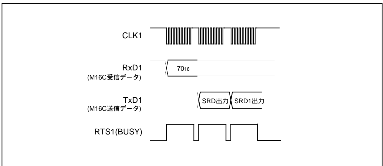
図1.25.3. リードステータスレジスタコマンド時のタイミング
