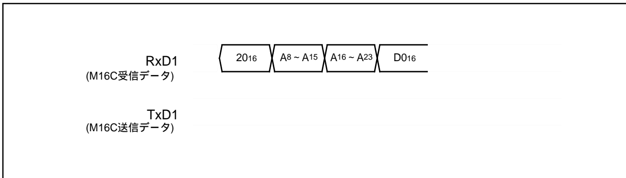
図1.25.26. ブロックイレーズコマンド時のタイミング
