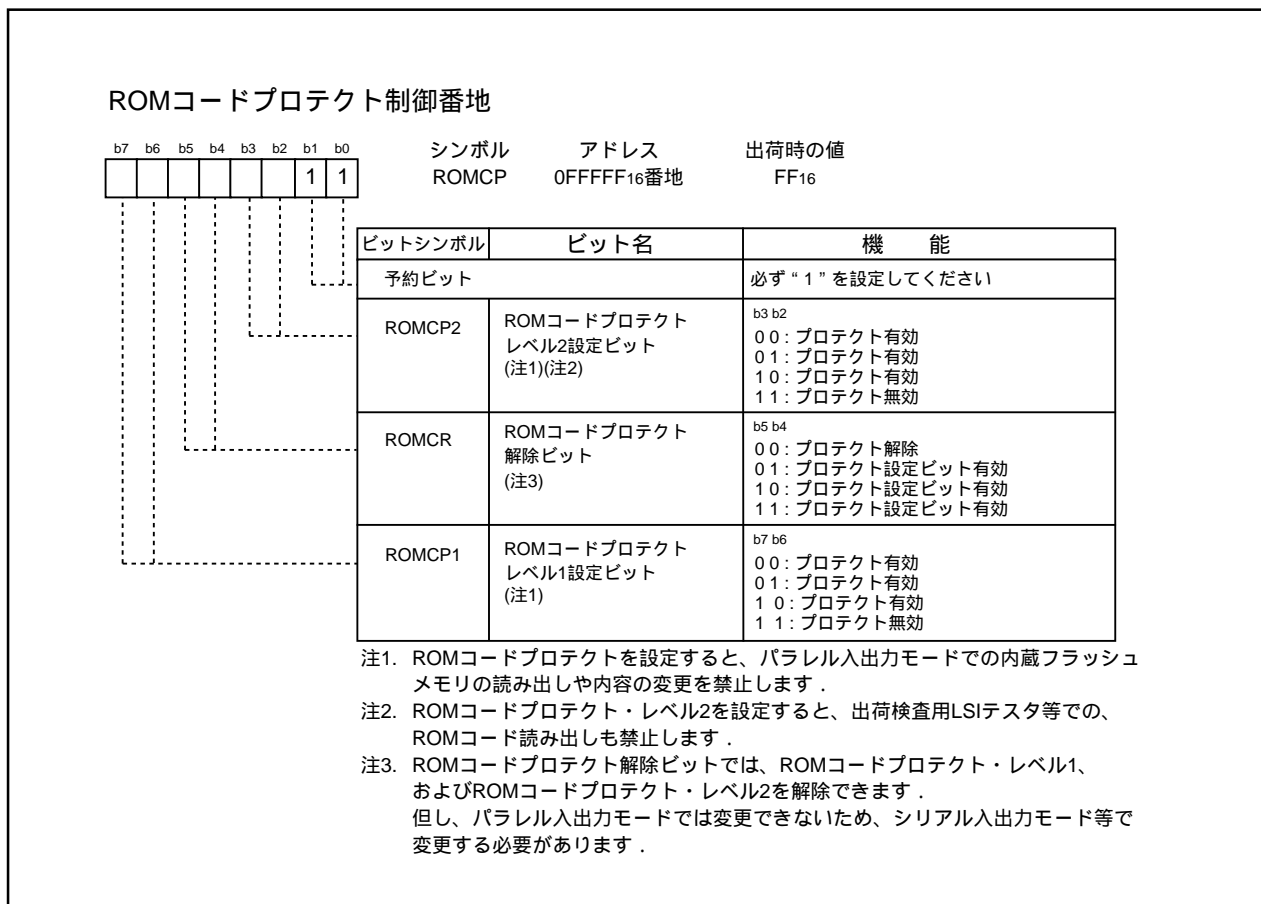
図1.23.1. ROMコードプロテクト制御番地の構成
