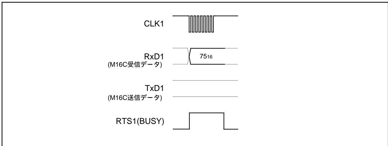
図1.25.11. ロックビット無効コマンド時のタイミング
