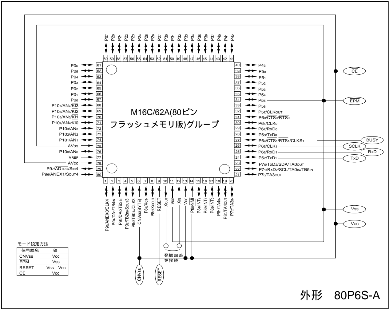
図1.25.1. 標準シリアル入出力モード時の端子結線図
