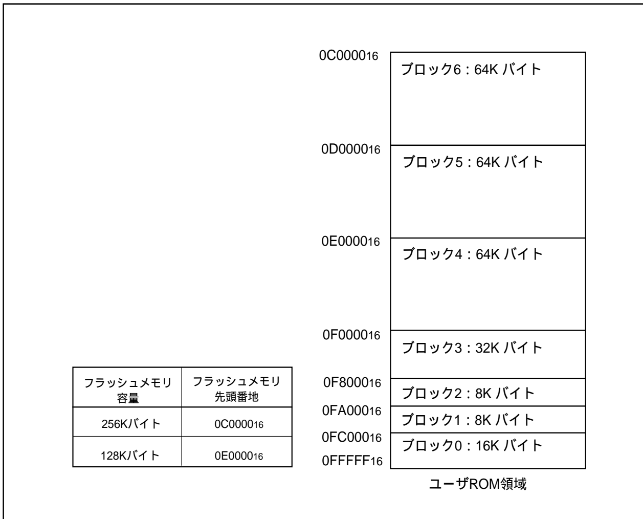
図1.25.18. ユーザ領域の各ブロック
