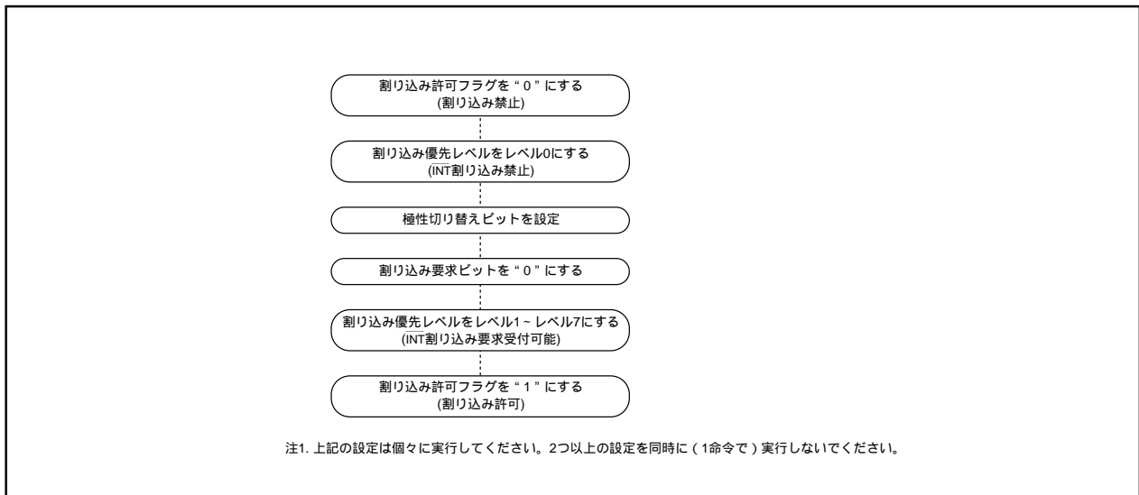
図1.10.13. INT割り込み発生要因の切り替え
