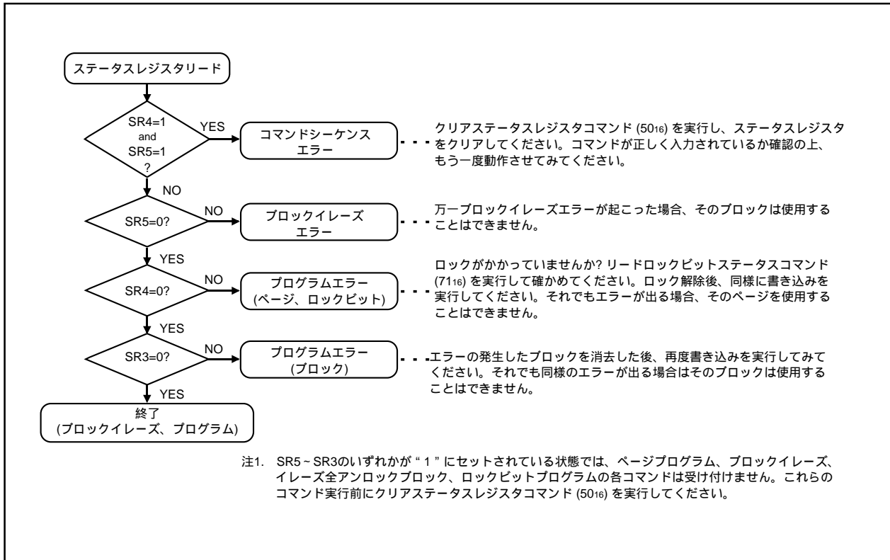
図1.25.19. フルステータスチェックフローチャートおよび各エラー発生時の対処法
