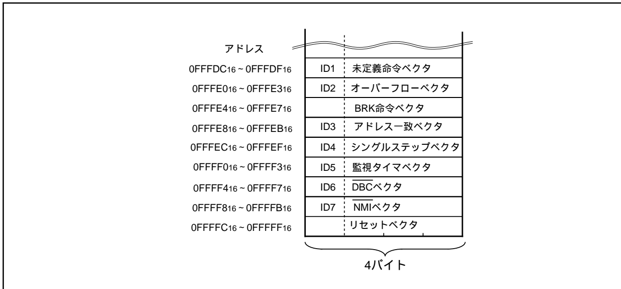
図1.23.2. IDコードの格納アドレス
