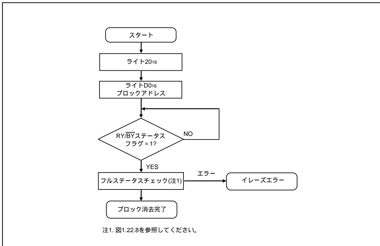
図1.22.5. ブロックイレーズフローチャート
