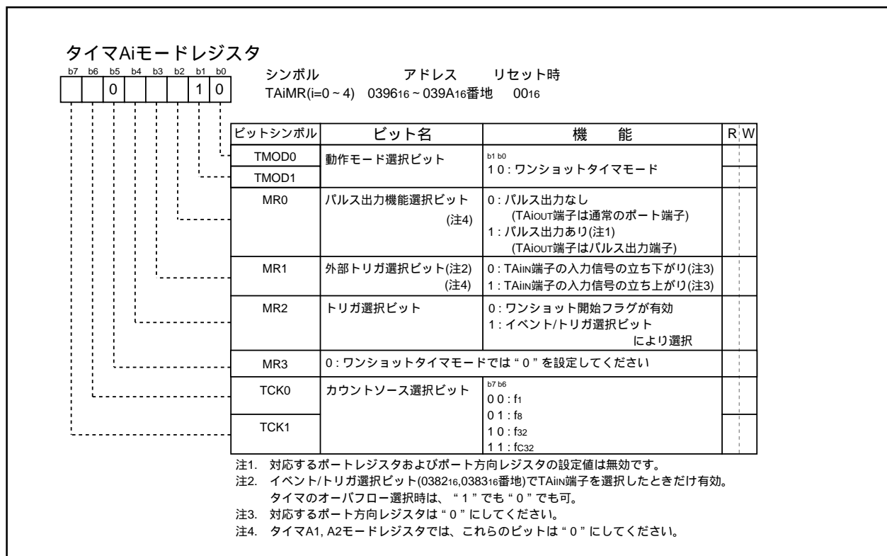
図1.13.10. ワンショットタイマモード時のタイマAiモードレジスタの構成
