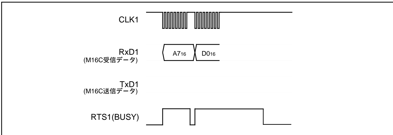
図1.25.7. イレーズ全アンロックブロックコマンド時のタイミング
