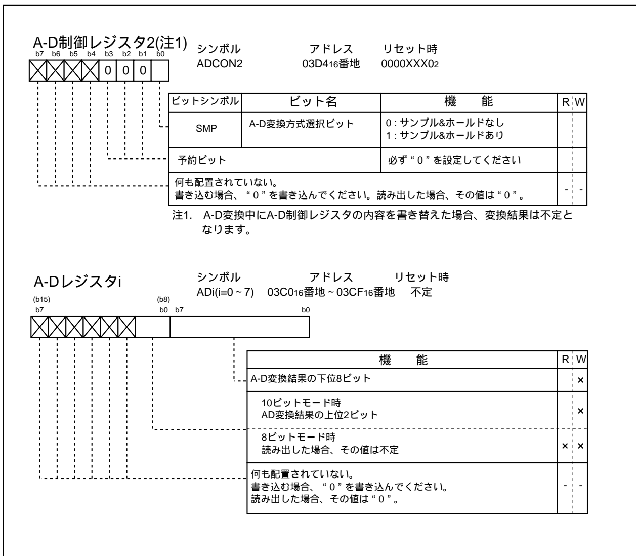
図1.15.3. A-D変換器関連レジスタ(2)
