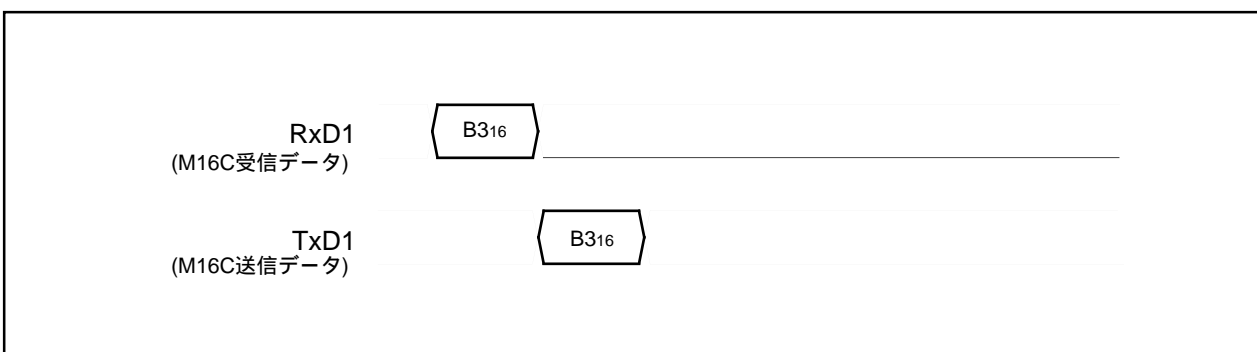
図1.25.41. ボーレート57600のタイミング
