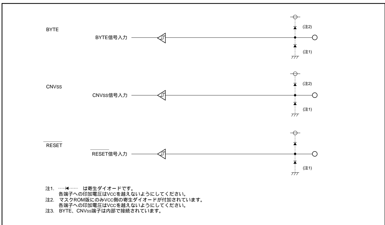
図1.18.5. 端子の構成
