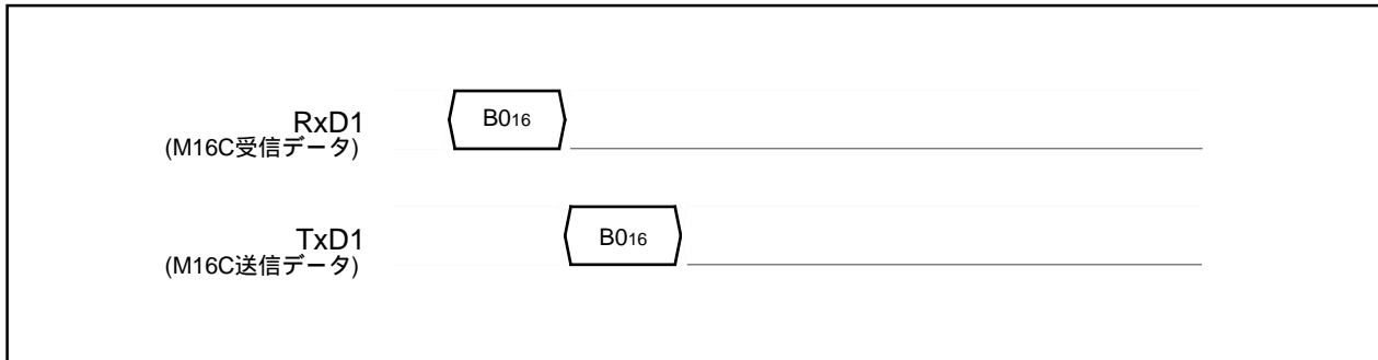
図1.25.38. ボーレート9600のタイミング
