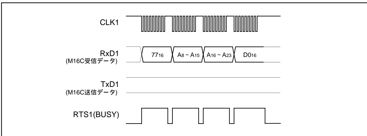
図1.25.8. ロックビットプログラムコマンド時のタイミング
