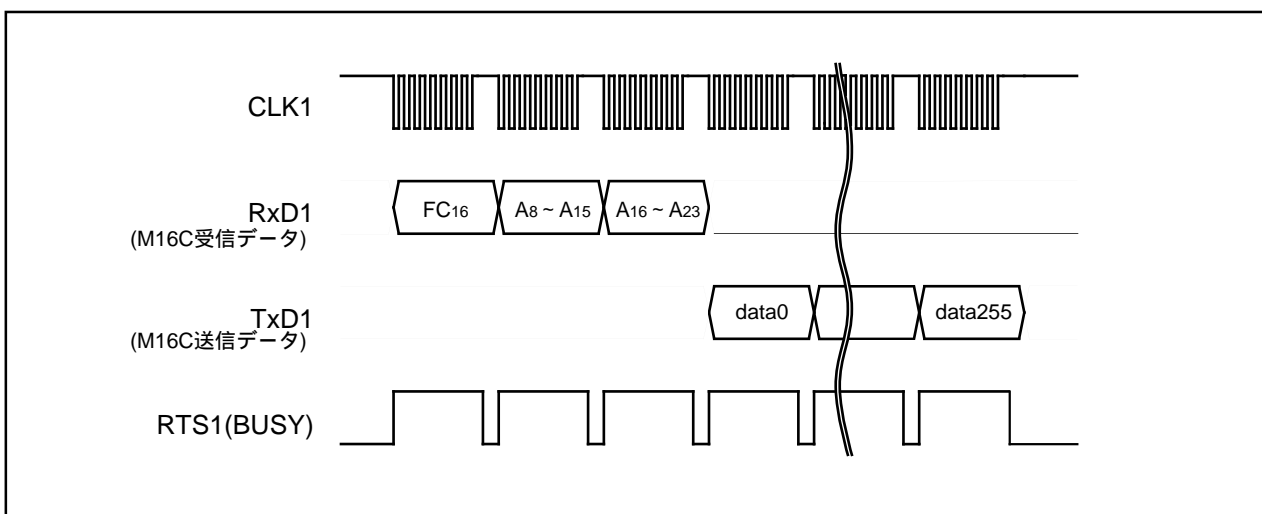
図1.25.14. ブートROM領域出力機能のタイミング
