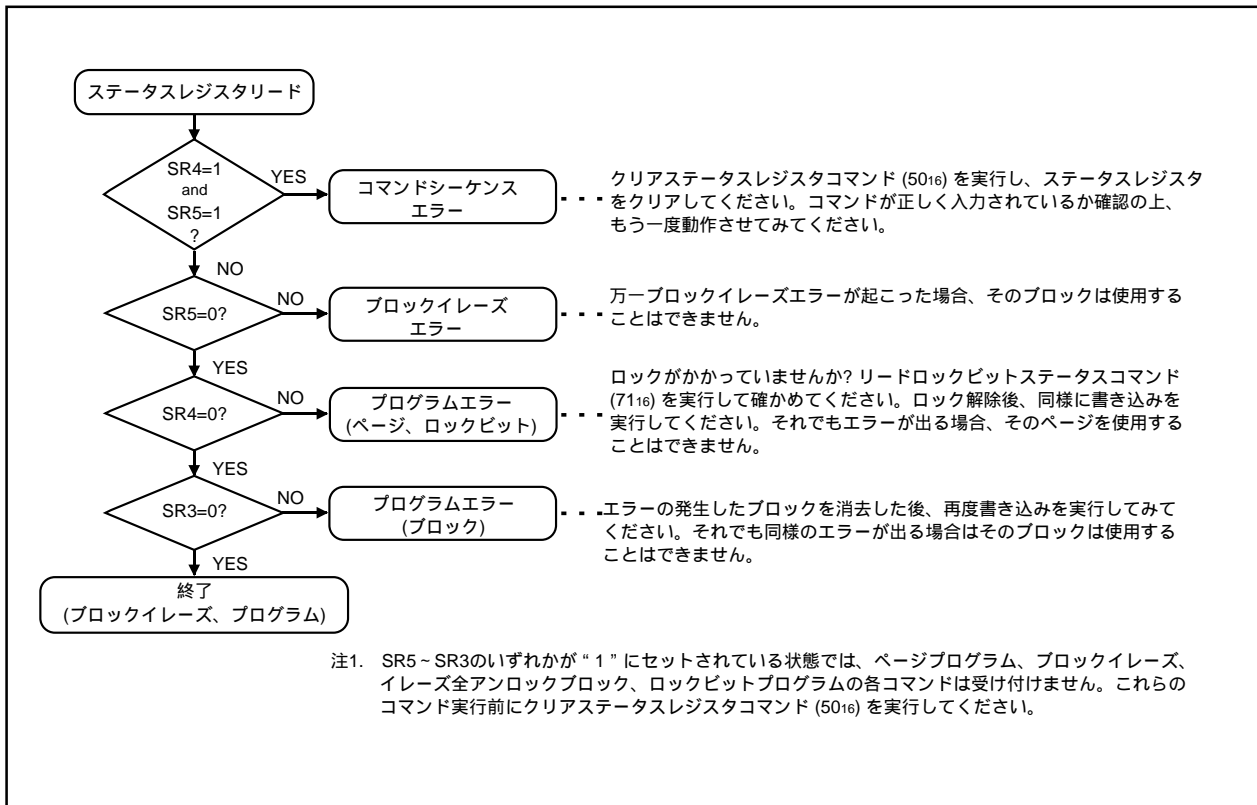
図1.22.8. フルステータスチェックフロチャートおよび各エラー発生時の対処方法
