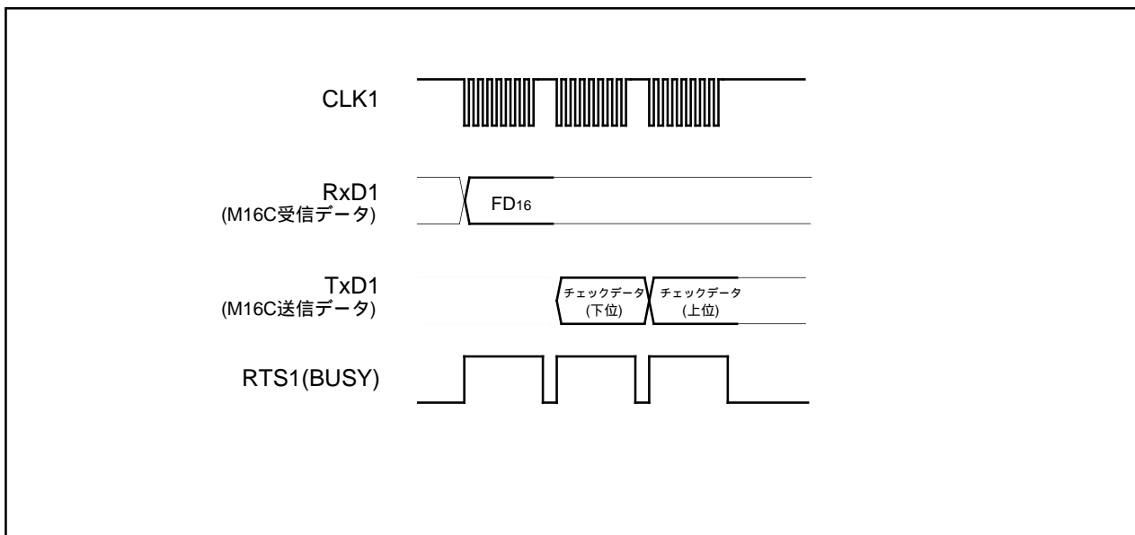
図1.25.17. リードチェックデータコマンド時のタイミング
