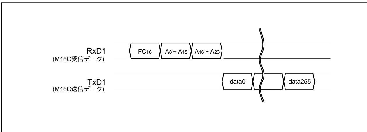
図1.25.34. ブートROM領域出力機能のタイミング
