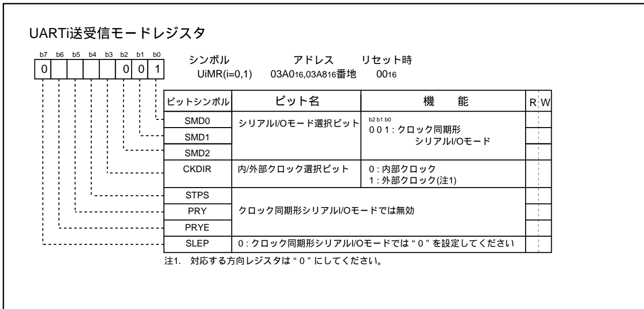
図1.14.10. クロック同期形シリアル/Oモード時のUART i 送受信モードレジスタの構成
