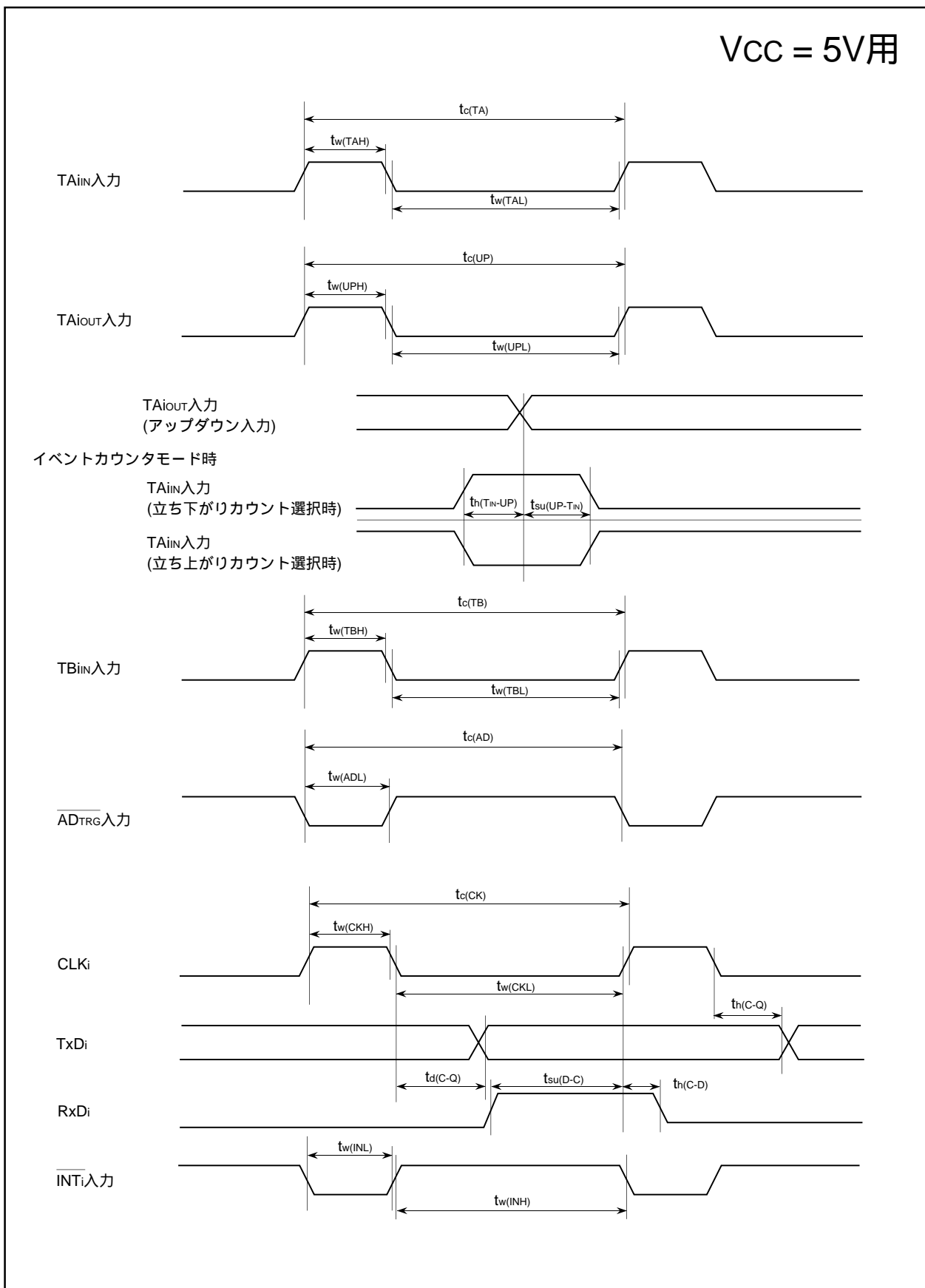
図1.20.1. VCC=5V用タイミング図
