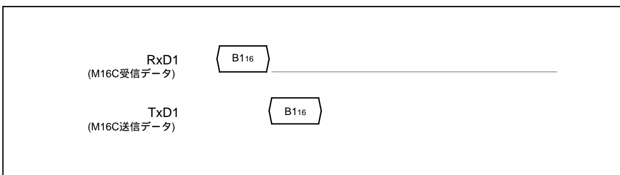
図1.25.39. ボーレート19200のタイミング
