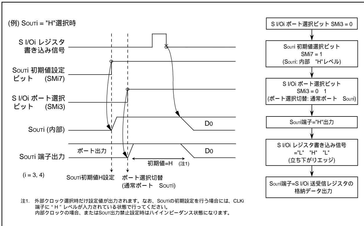
図1.14.32. Sout i 初期値設定 タイミング図および設定方法
