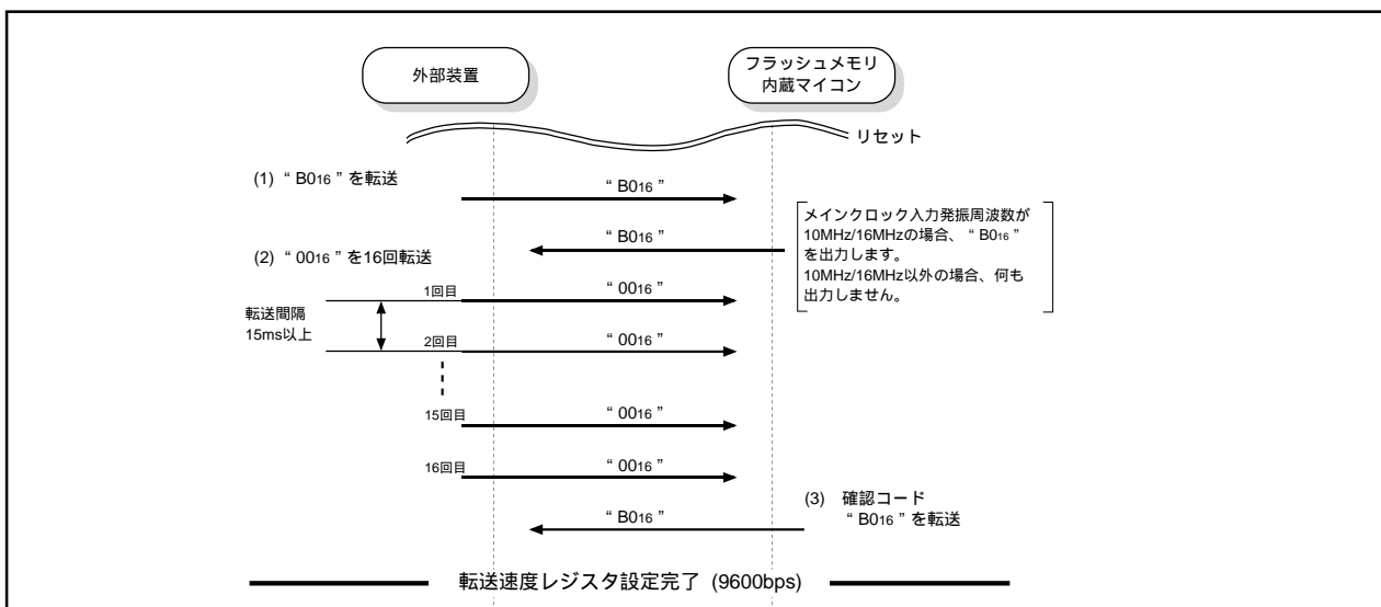
図1.25.21. 外部装置との初期通信
