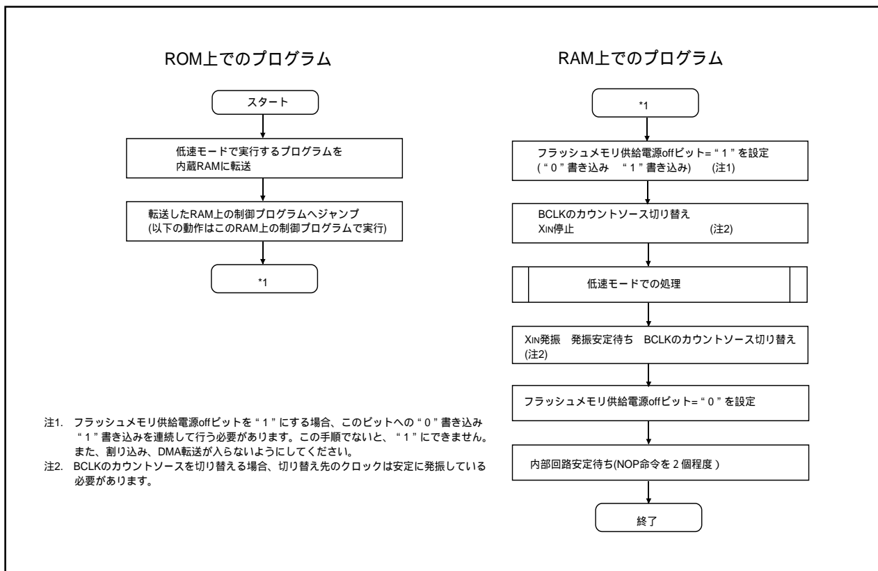
図1.22.3. 低速モードを実現するためのフローチャート
