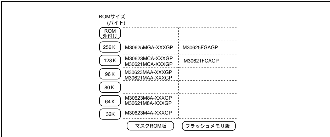
図1.1.3. ROM展開
