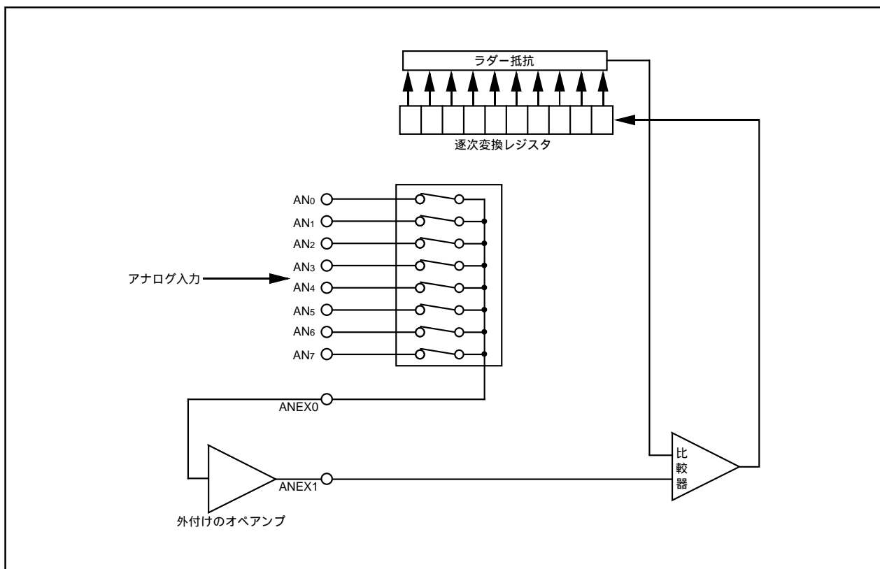
図1.15.9. 外部オペアンプ接続モードの接続例
