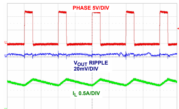
図 13. フル負荷時の定常状態動作 ( 1\mu\text{s}/\text{DIV} )
