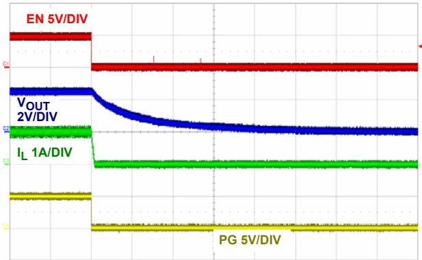
図 17. シャットダウン回路 (100 \mu\text{s} /DIV)
