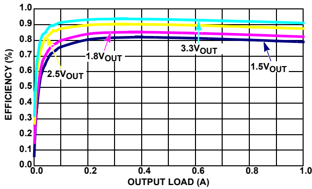
図 2. 効率 vs 負荷、500kHz、5V IN
