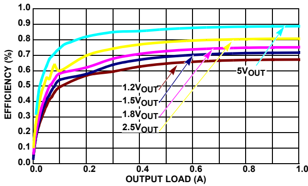
図 4. 効率 vs 負荷、500kHz、25V IN
