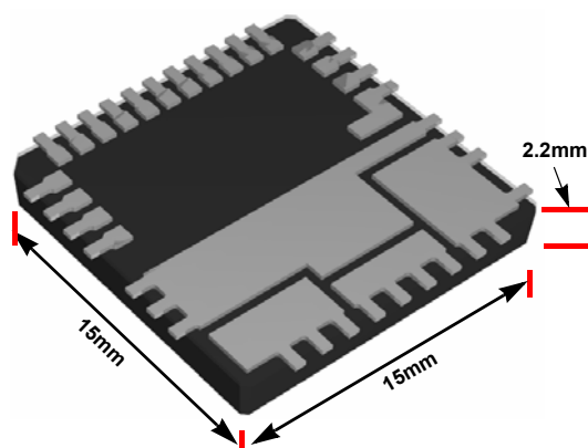
図 2. 2.2mm と低背なため、面積や高さが限られている場合に PCB 裏面への実装が可能
