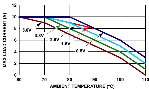
図 40. ディレーティング曲線 (12V IN )、出力電圧別に OLFM で測定
