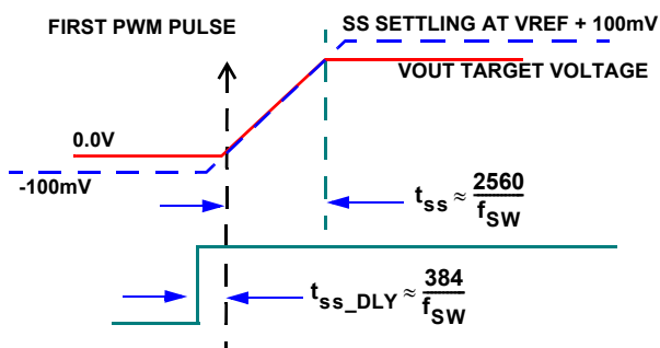
図 26. V_{OUT} = 0V の場合のソフトスタート
