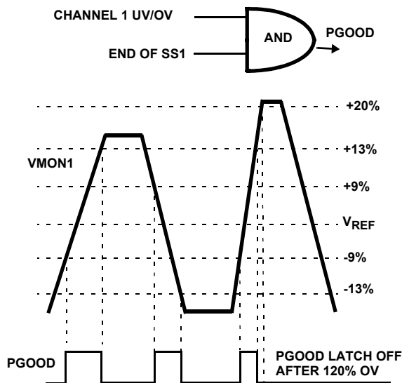
図 30. パワーグッド・スレッショルド・ウィンドウ
