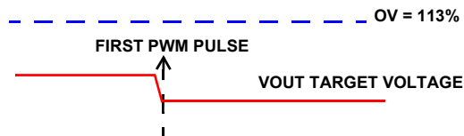
図 28. V_{OUT} が OV より低く最終目標電圧より高い場合のソフトスタート
