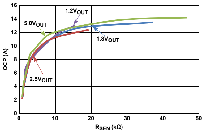
図 32. 12V IN
