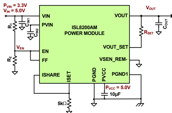
図 21. 3.3V での動作
