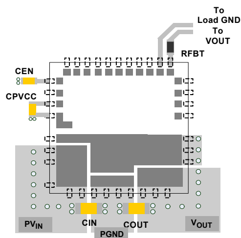
図 35. シングルフェーズ・セットアップの推奨レイアウト
