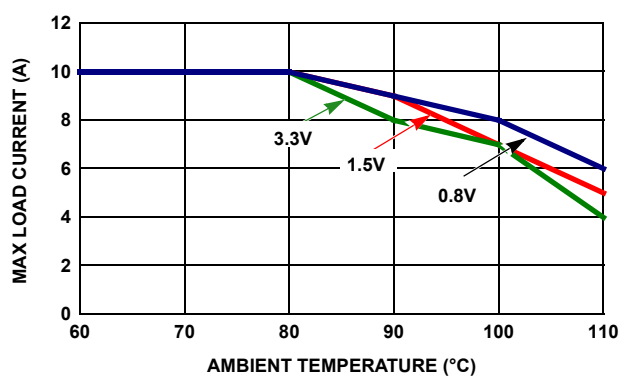
図 38. ディレーティング曲線 (5V IN )、出力電圧別に OLFM で測定
