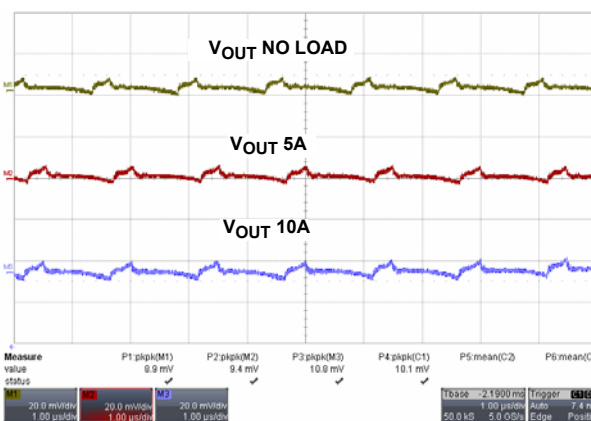
図 19. 2.5V 出力リップル
