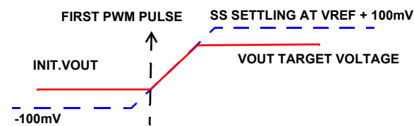
図 27. V_{OUT} < \text{目標電圧} の場合のソフトスタート
