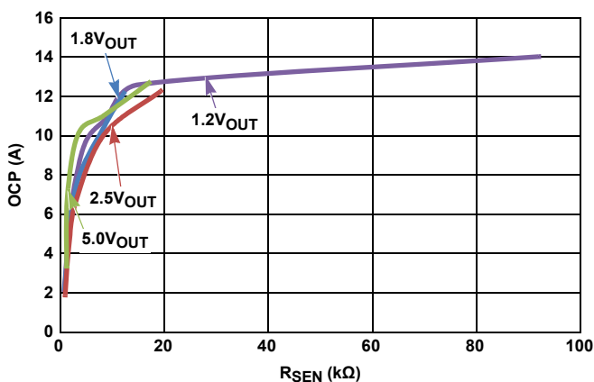
図 33. 20V IN
