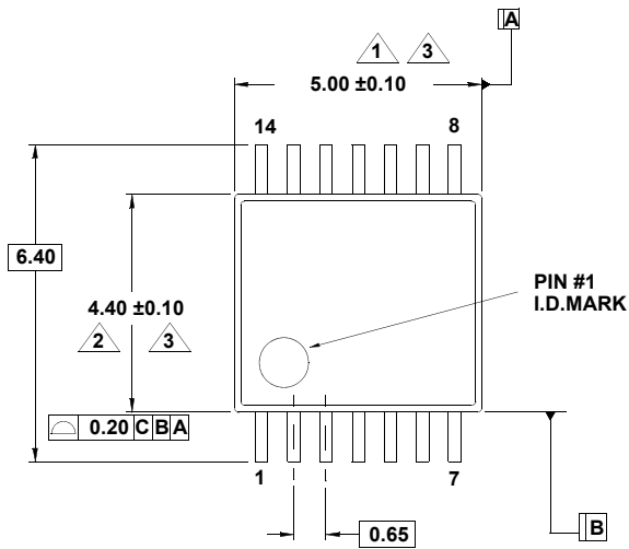
上面図
