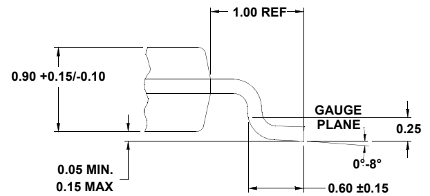
"X"の詳細
