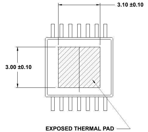
底面図
