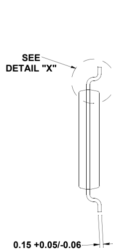
端面図
