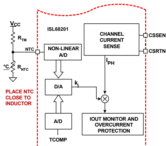
図 17. 内蔵温度補償のブロック図
