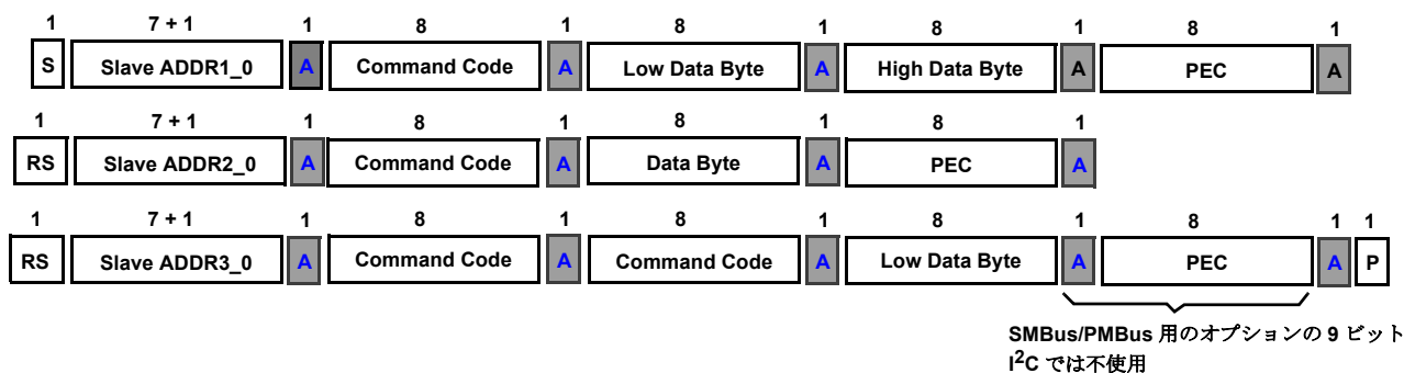
図 24. SMBus/PMBus/I 2 C コマンドのプロトコル
