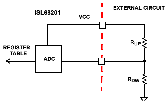
図 6. 単純化された分割抵抗 ADC
