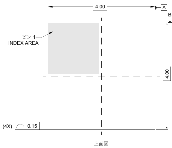
上面図
