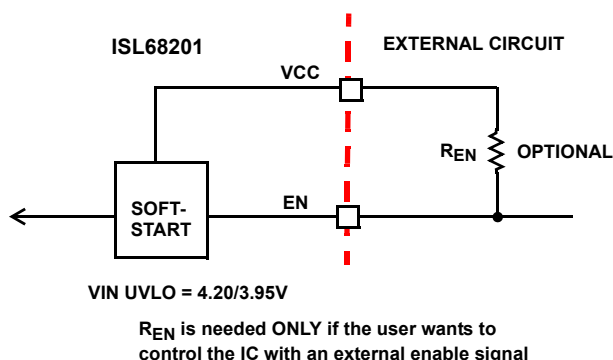
図 5. 5V 入力または広範囲の入力の構成
