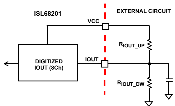
図 20. I_{OUT} の無負荷オフセットの校正
