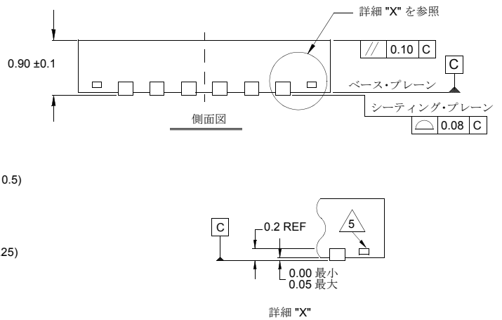
詳細 "X"
