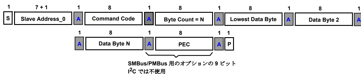
図 23. SMBus/PMBus/I²C コマンドのプロトコル
