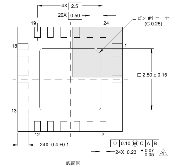
底面図
