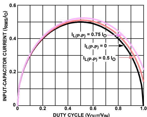
図 30. 正規化された入力コンデンサの RMS 電流と、 シングルフェーズ・コンバータの デューティ・サイクルとの関係
