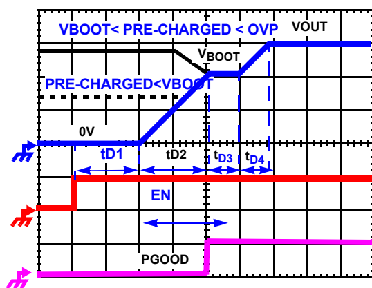
図 7. ソフトスタートの波形
