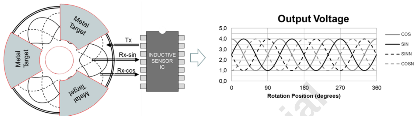
図 30 3 × 120° ロータリセンサ用のコイル設計と信号出力
