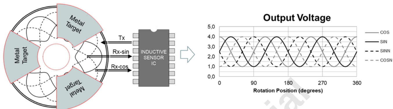
図 30 3 \times 120^\circ ロータリセンサ用のコイル設計と信号出力
