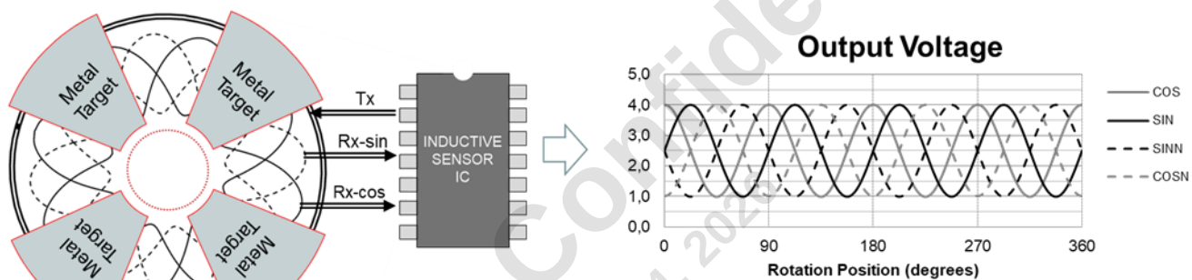
図 31 4 × 90° ロータリセンサ用のコイル設計と信号出力
