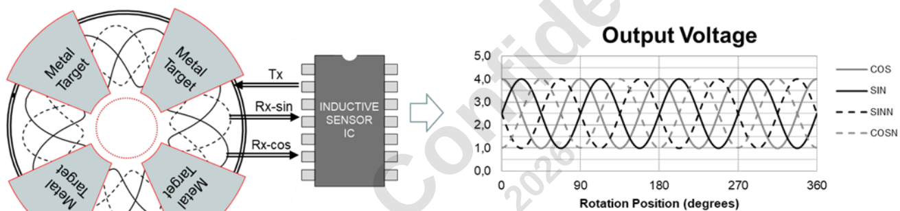
図 31 4 \times 90^\circ ロータリセンサ用のコイル設計と信号出力
