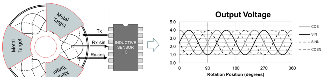
図 30 3 \times 120^\circ ロータリセンサ用のコイル設計と信号出力
