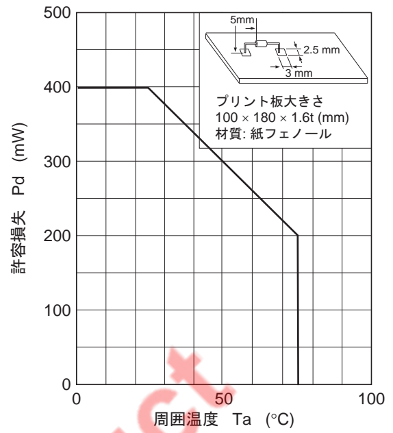
図2. 許容損失 対 周囲温度特性
