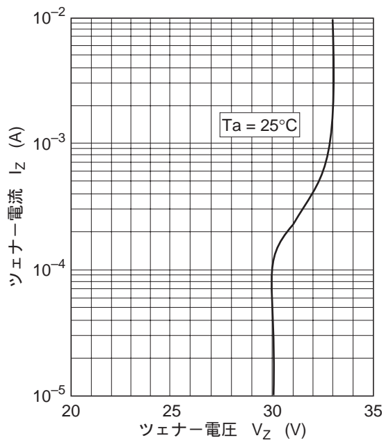
図1. ツェナー電流 対 ツェナー電圧特性
