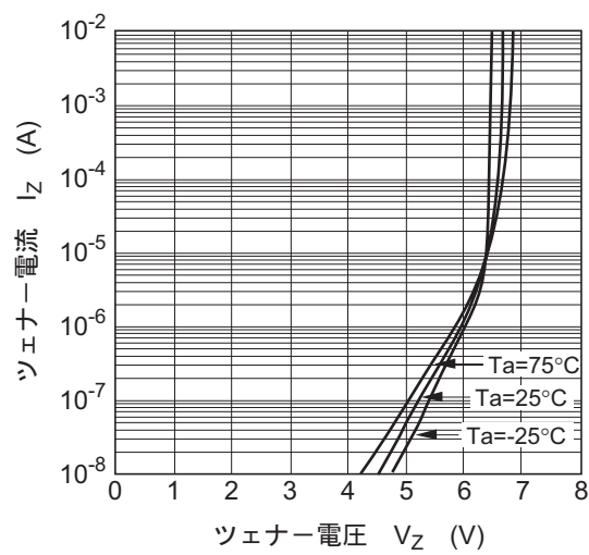
図1. ツェナー特性
