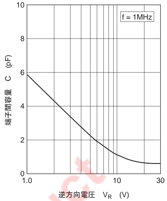
图2. 端子間容量 对 逆电压特性
