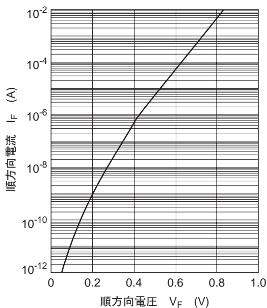
图1. 顺方向特性
