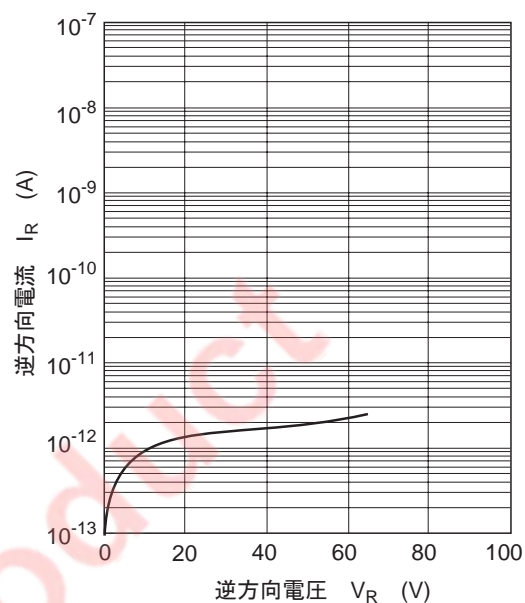
图2. 逆方向特性
