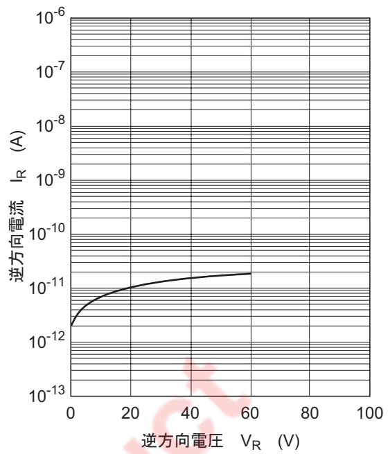
图2. 逆方向特性
