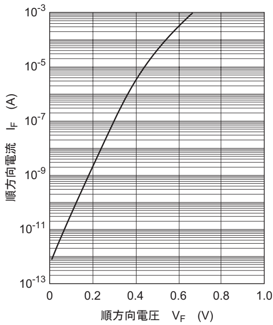
图1. 顺方向特性
