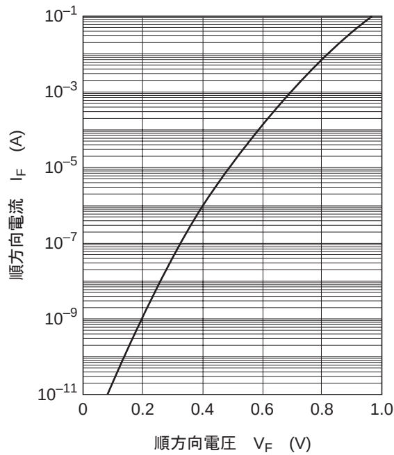
图1. 順方向特性
