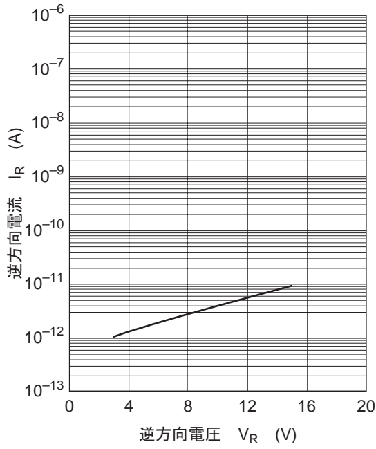
图1. 逆方向特性
