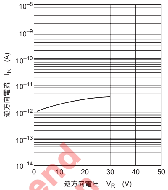
图2. 逆方向特性
