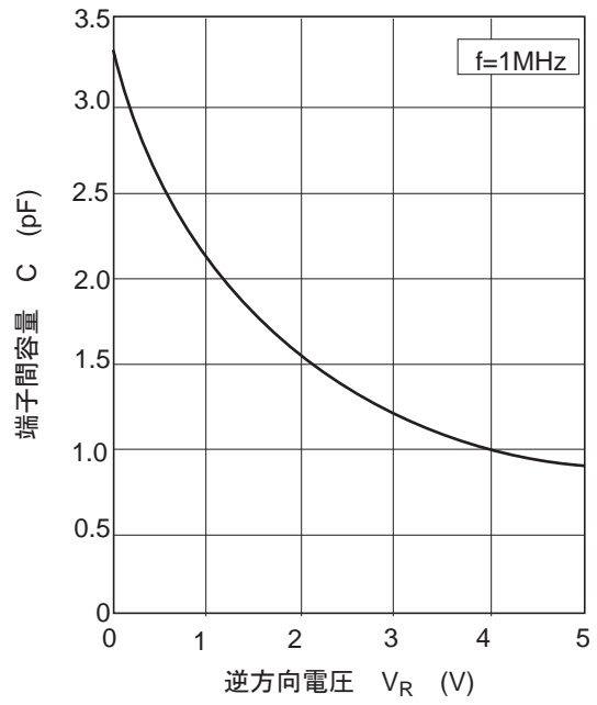
図2. 端子間容量 対 逆電圧特性
