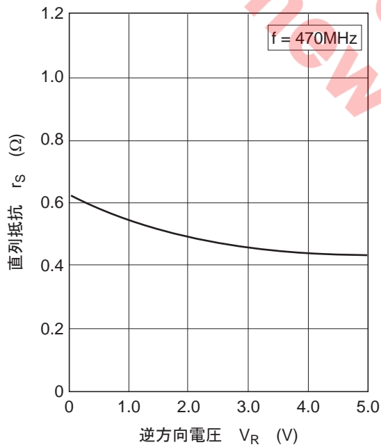
図3. 直列抵抗 対 逆電圧特性
