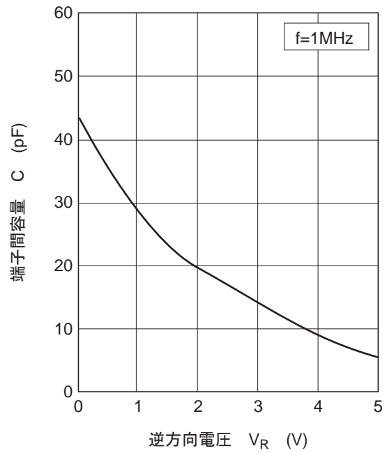
図2. 端子間容量 对 逆电压特性
