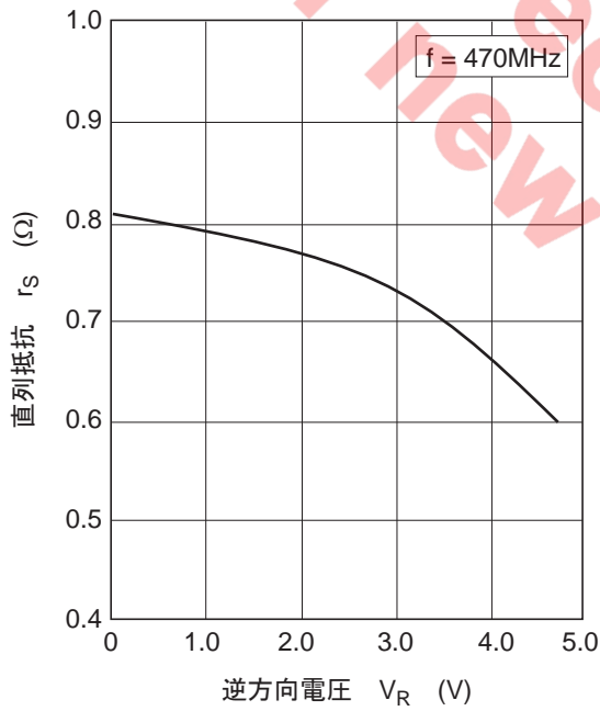
図3. 直列抵抗 对 逆电压特性
