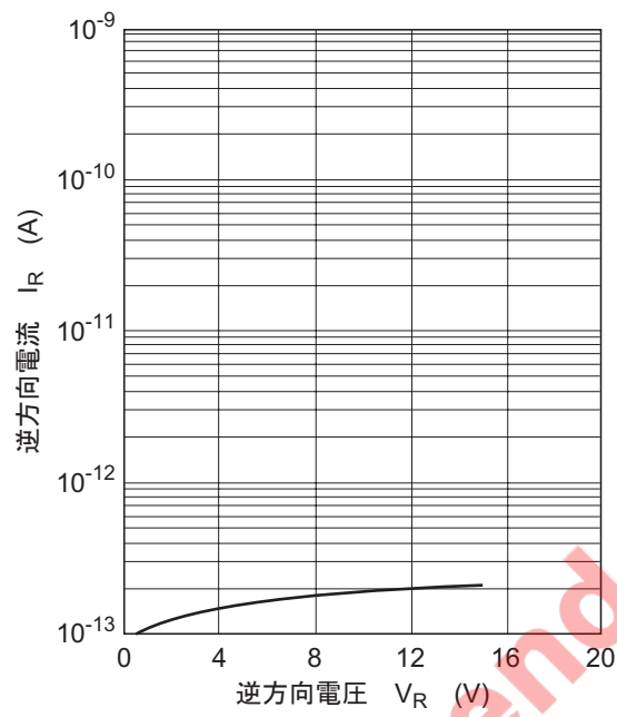
図1. 逆方向特性
