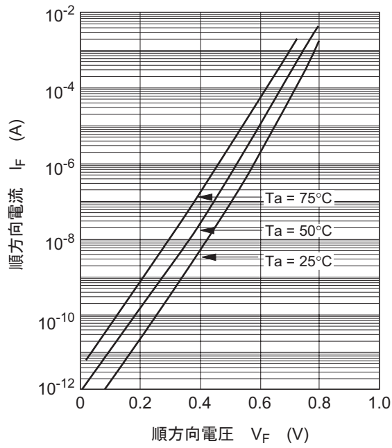
图1. 顺方向特性
