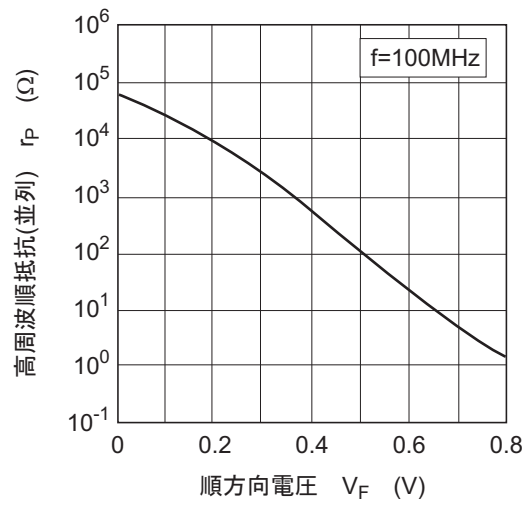
图5. 高周波順抵抗(並列) 对 順電圧特性
