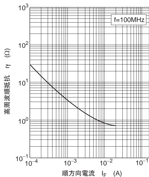
图4. 高周波顺抵抗 对 顺电流特性
