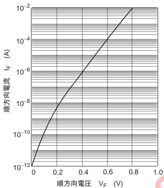
图1. 顺方向特性
