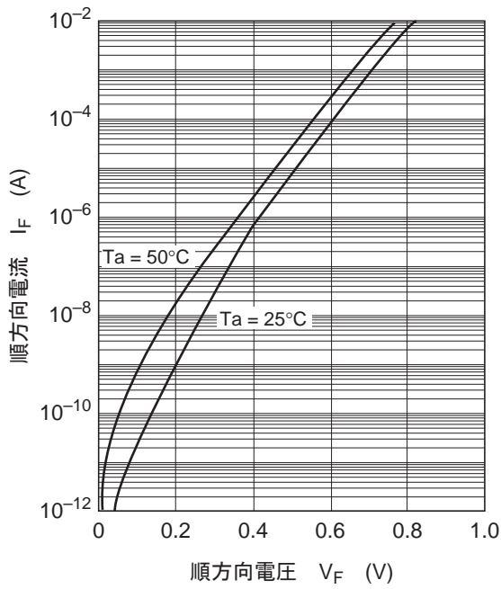
图1. 顺方向特性
