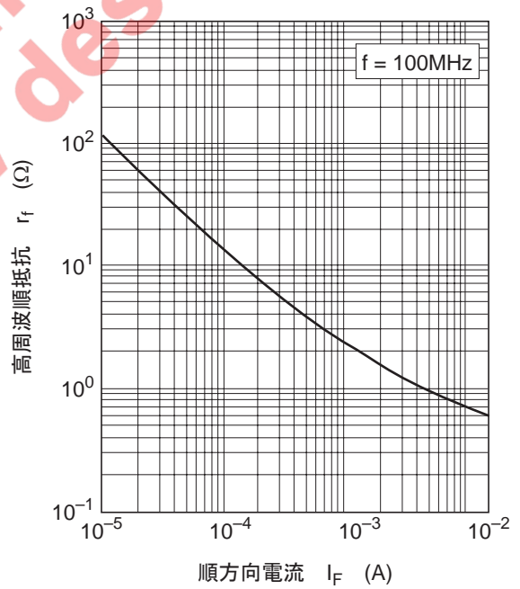
图4. 高周波顺抵抗 对 顺电流特性
